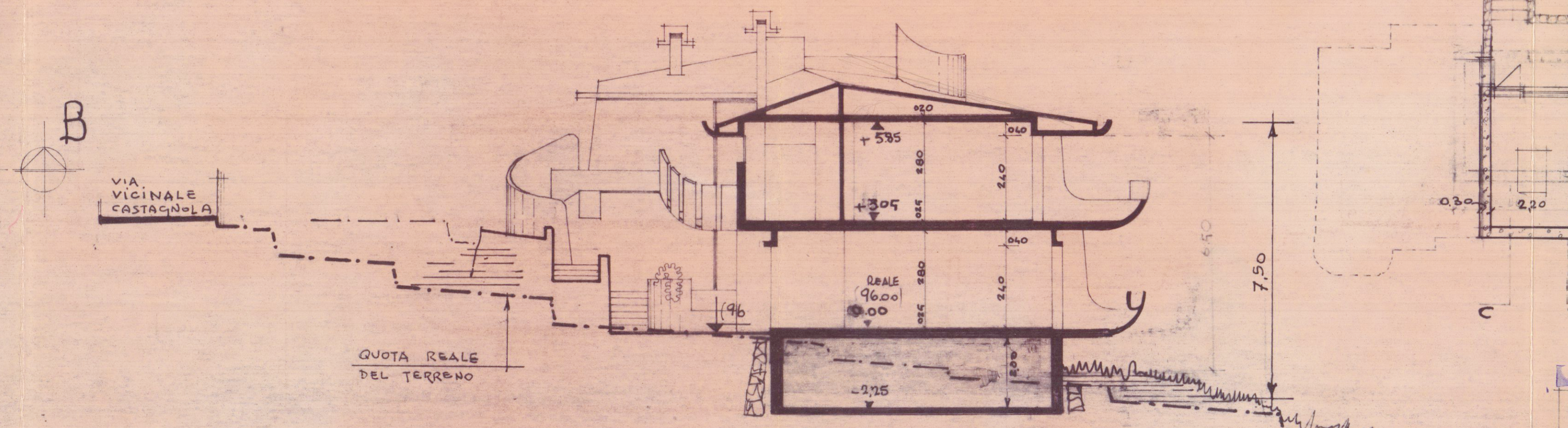
SEZIONE A.A.
