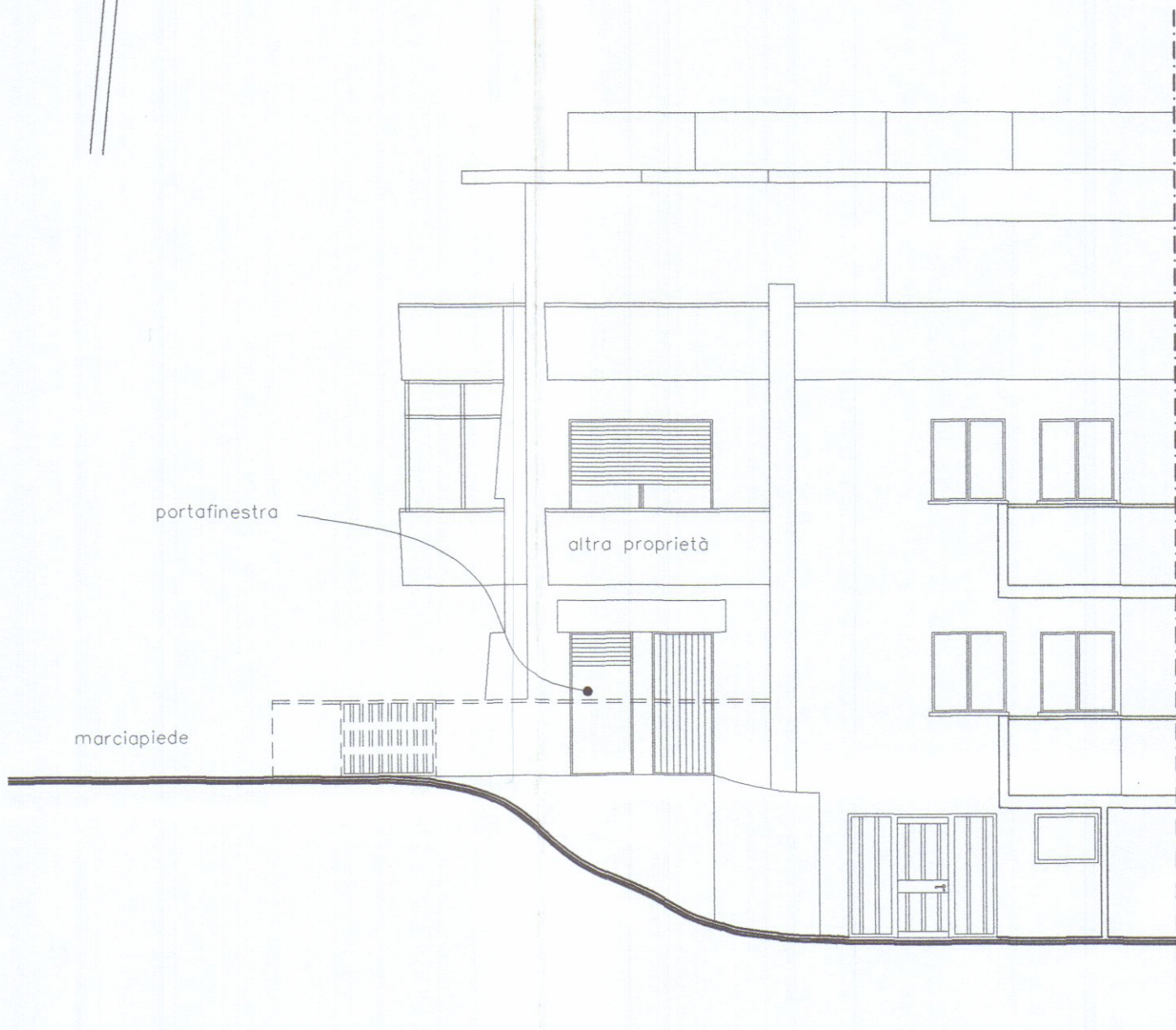
PROSPETTO EST
