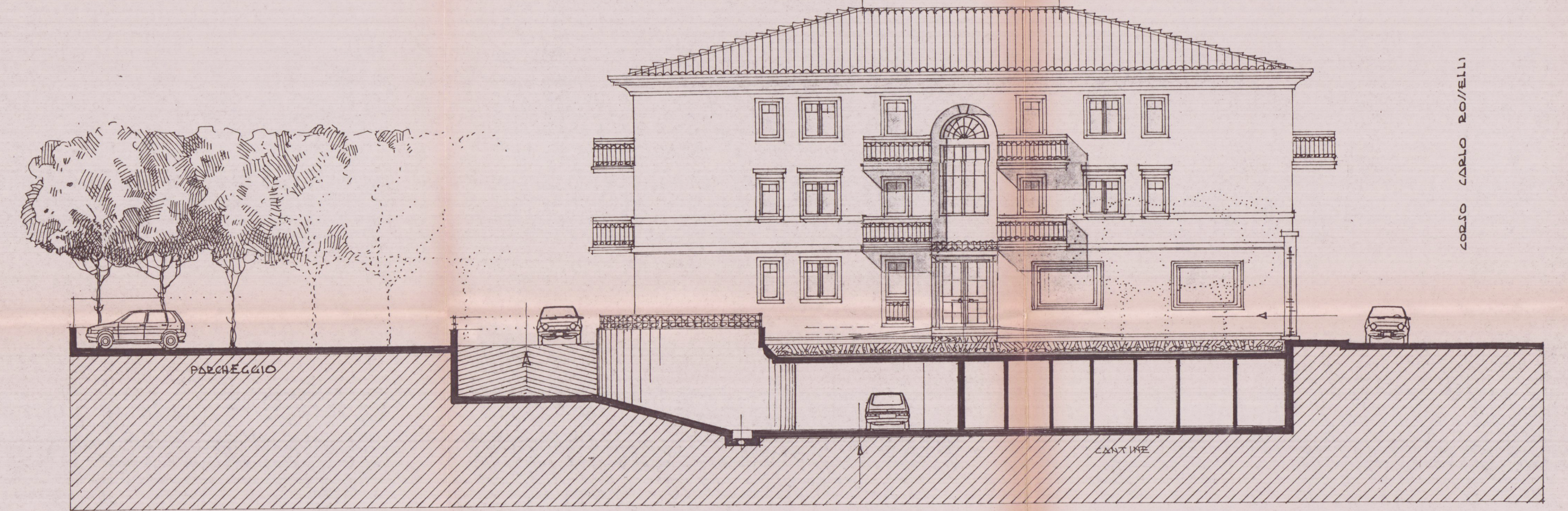
PROSPETTO SUD
