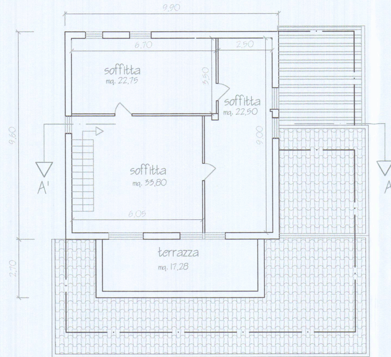
PIANO SOTTOTETTO
