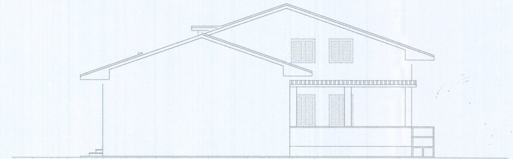
PROSPETTO EST
