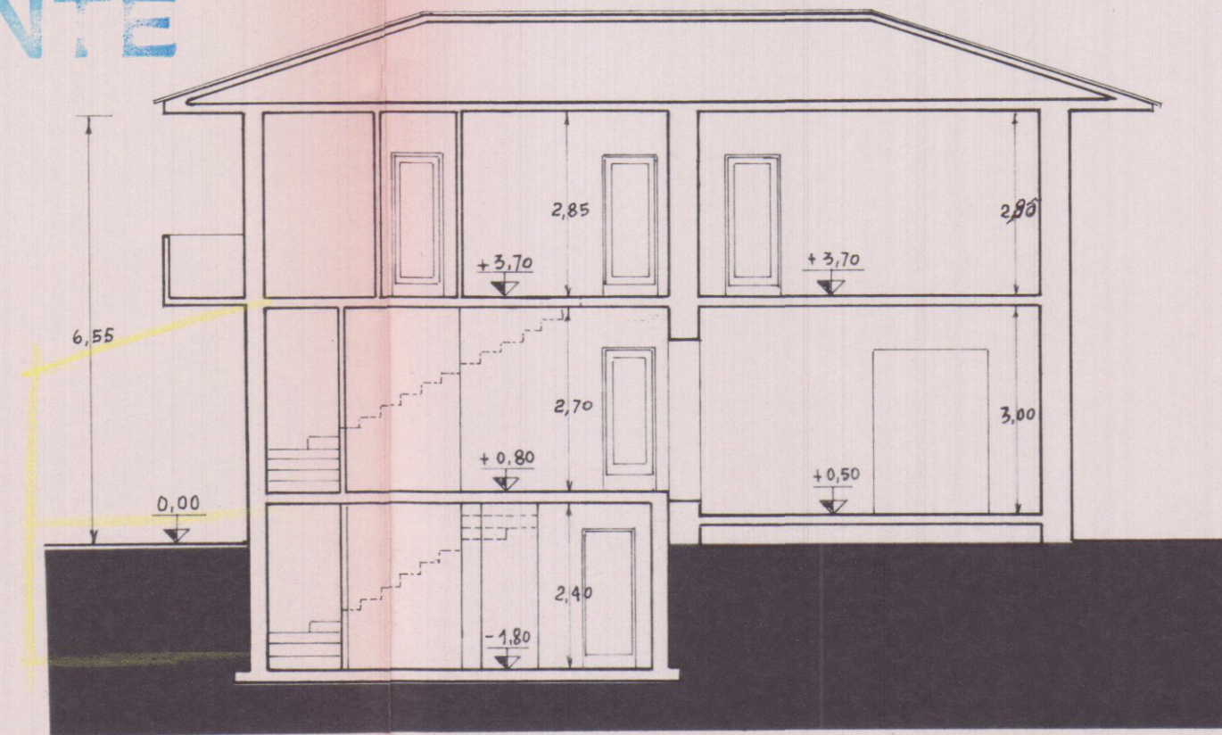
SEZIONE A-A
