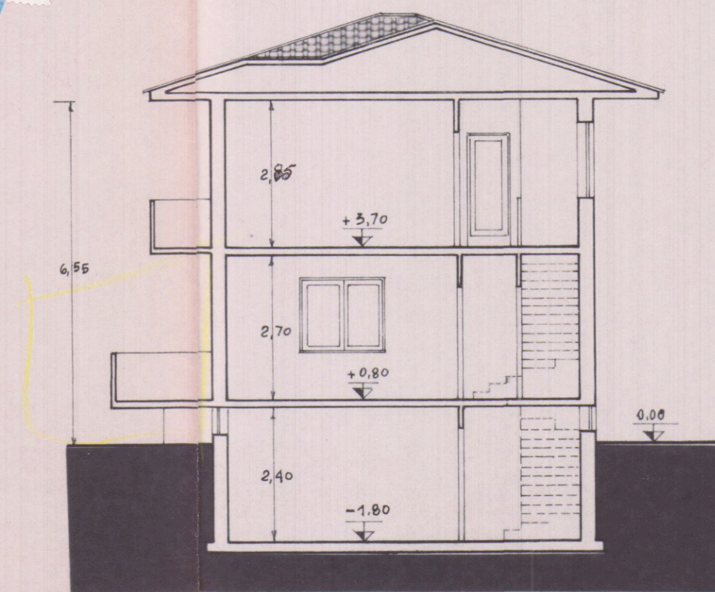
SEZIONE B-B
