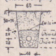
SEZIONE TRASVERSALE (in terreno compatto)
