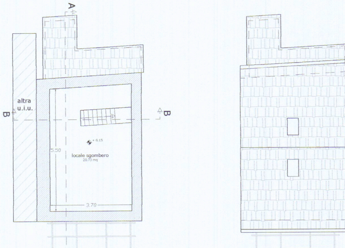
Piano Sottotetto
