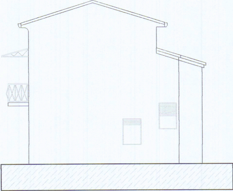
Prospetto Nord-Est
