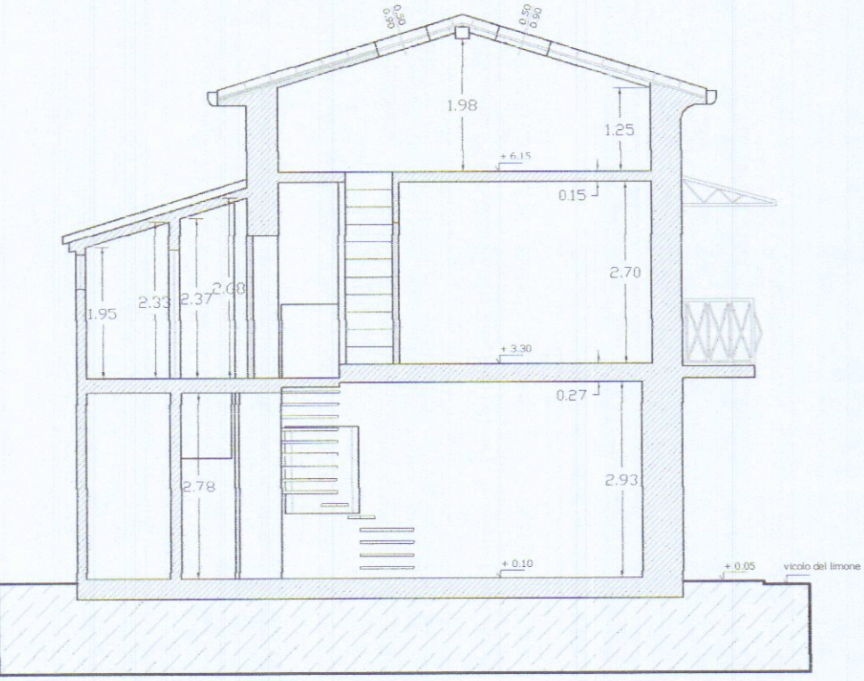
Sezione A-A
