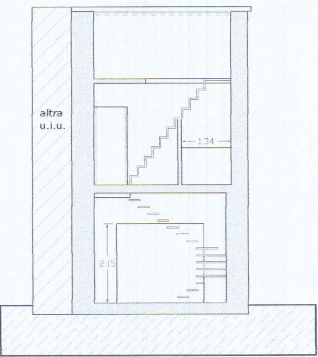
Sezione B-B
