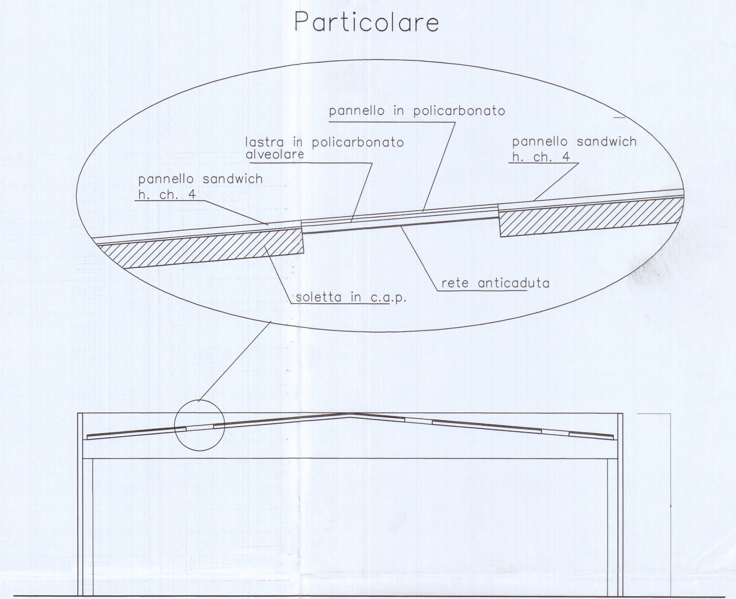
Sezione A-A'
