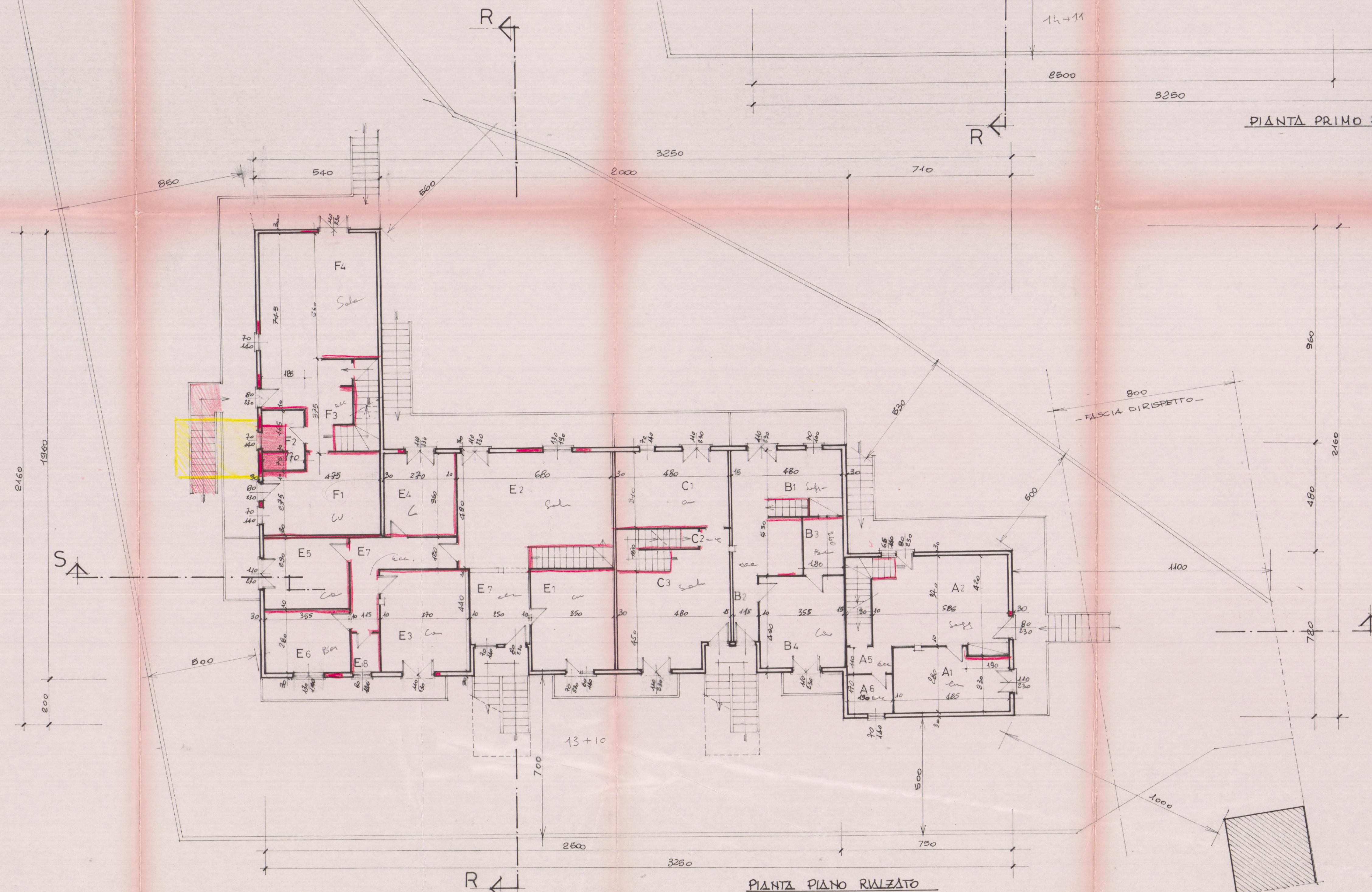
PIANTA PIANO REALIZZATO
