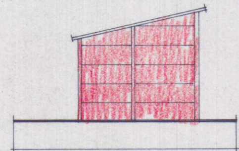
PROSPETTO LATO S.E.
