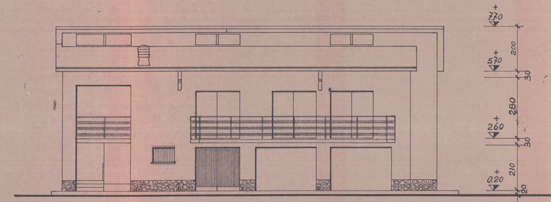
FACCIATA VERSO MARE (SUD)
