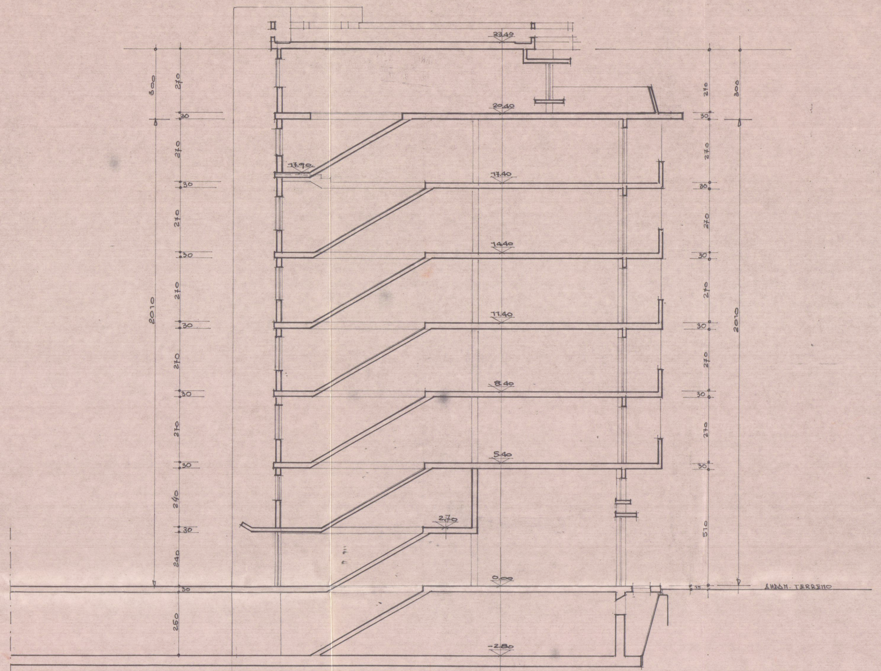
SEZIONE TRASVERSALE
