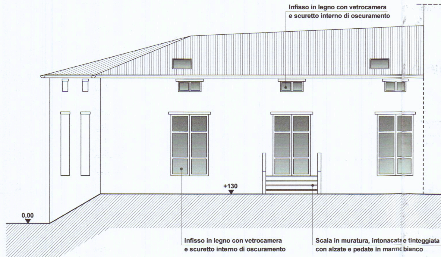
PROSPETTO POSTERIORE
