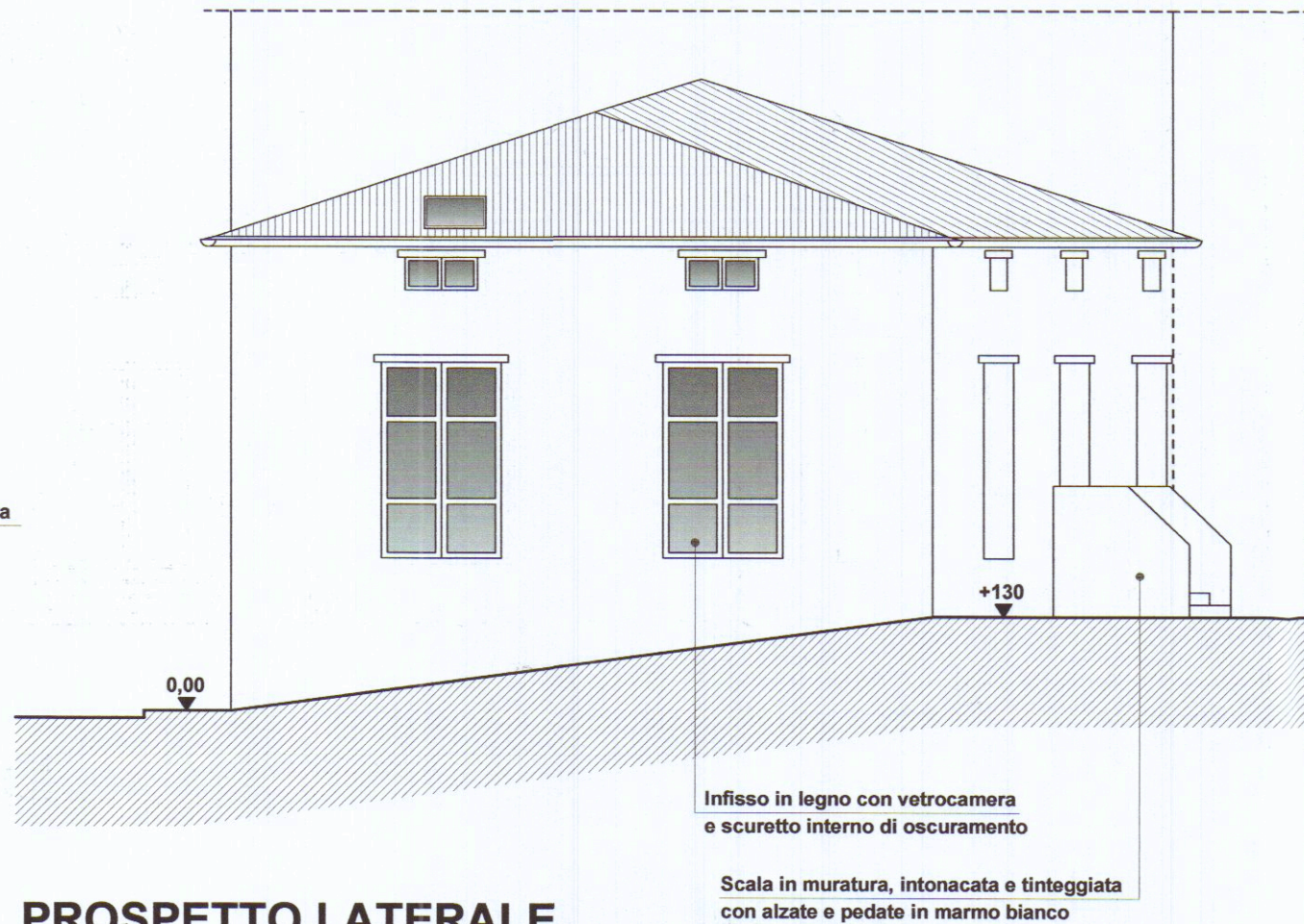
PROSPETTO LATERALE
