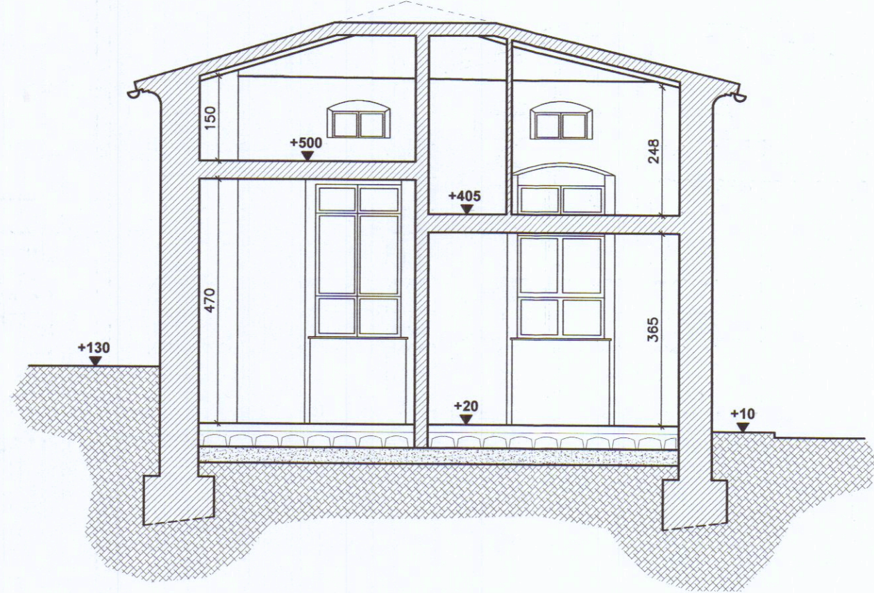
SEZIONE S01
