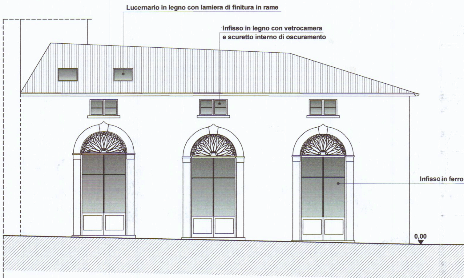
PROSPETTO PRINCIPALE
