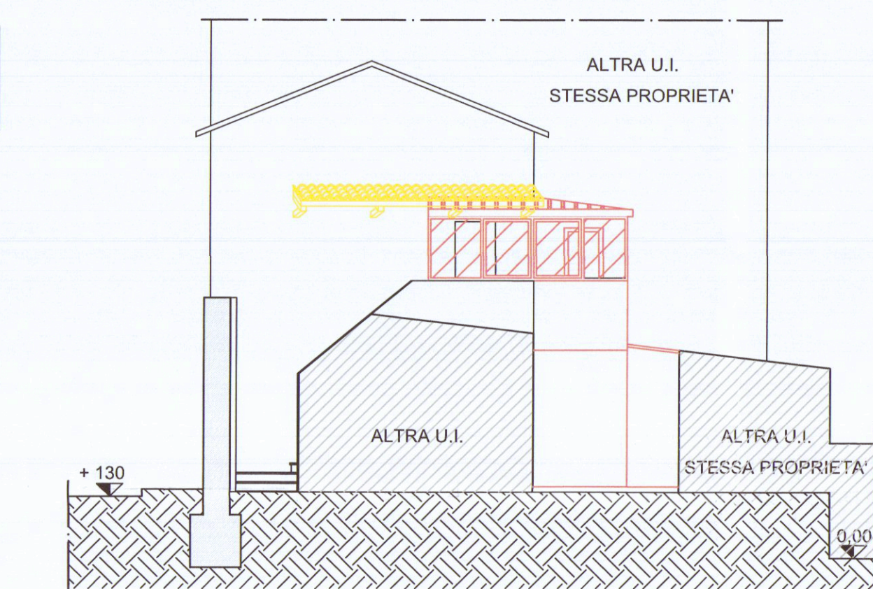
PROSPETTO OVEST
