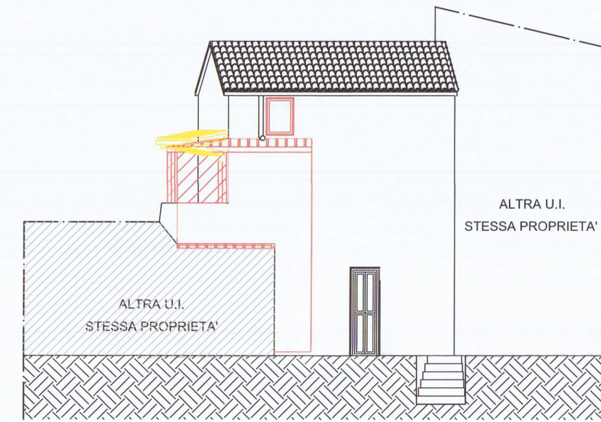
PROSPETTO SUD OVEST
