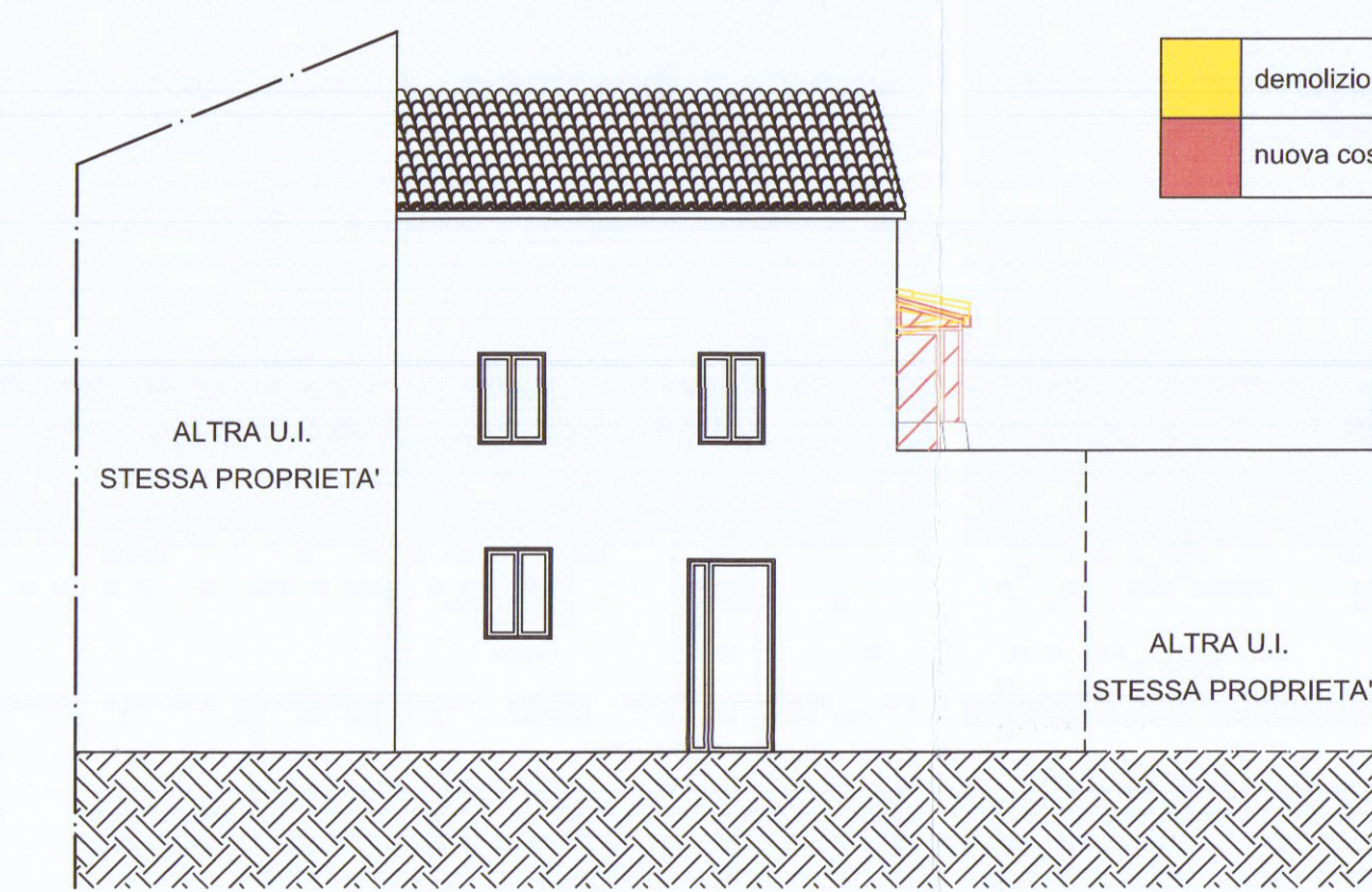
PROSPETTO NORD EST
