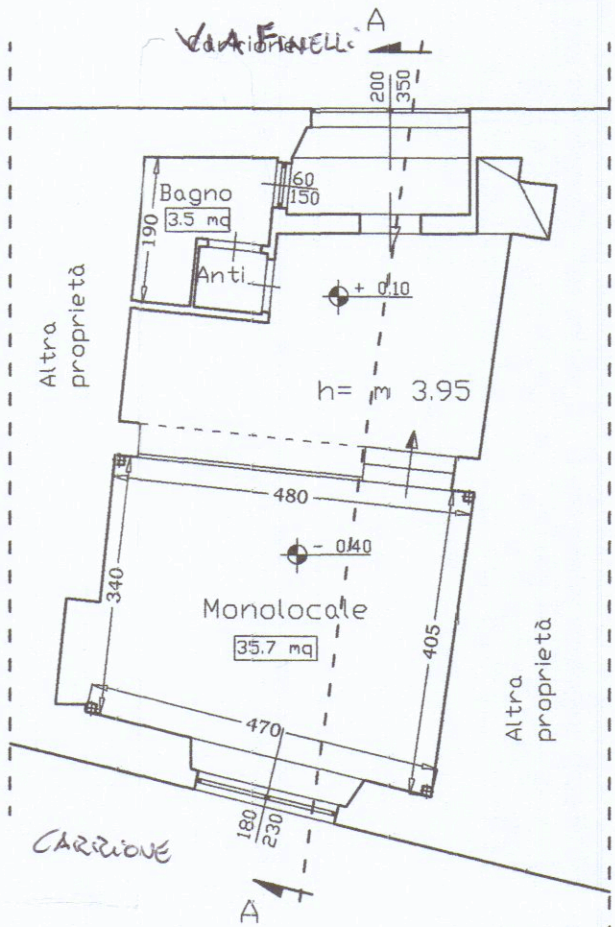
PIANTA PIANO TERRA (progetto)
