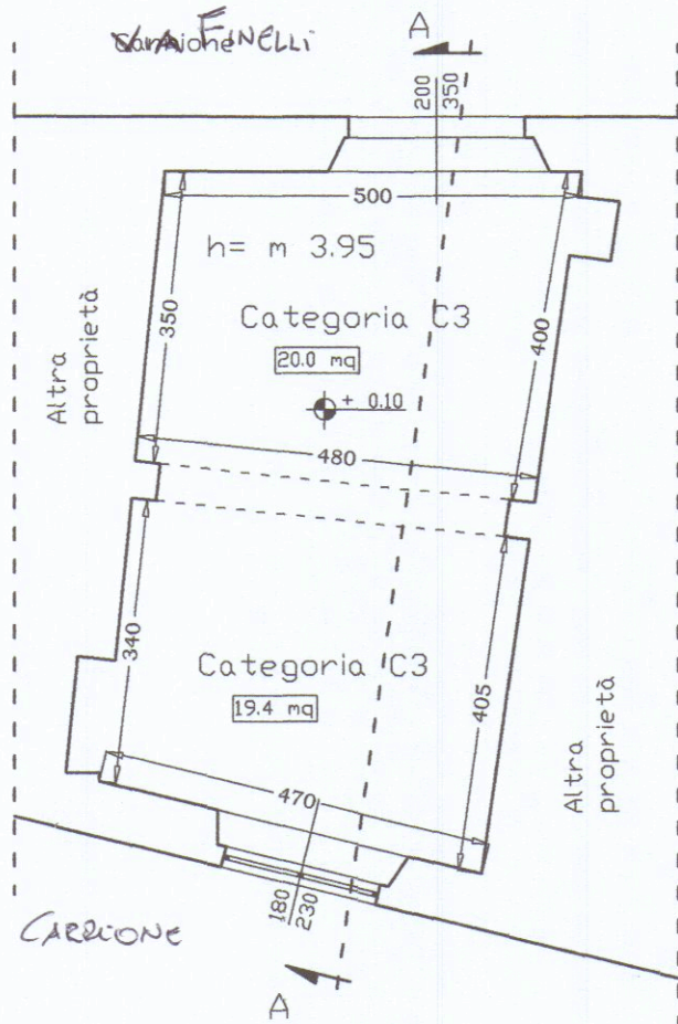
PIANTA PIANO TERRA (esistente)
