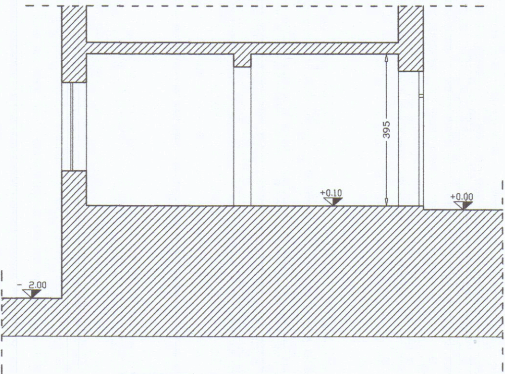
SEZIONE A-A (esistente)
