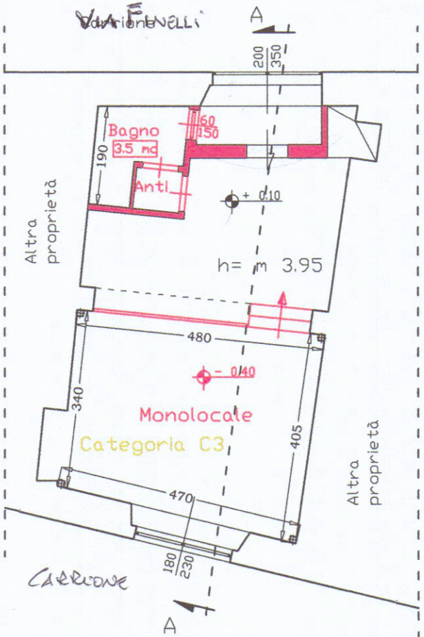
PIANTA PIANO TERRA (raffronto)
