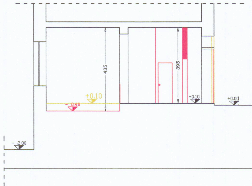
SEZIONE A-A (raffronto)
