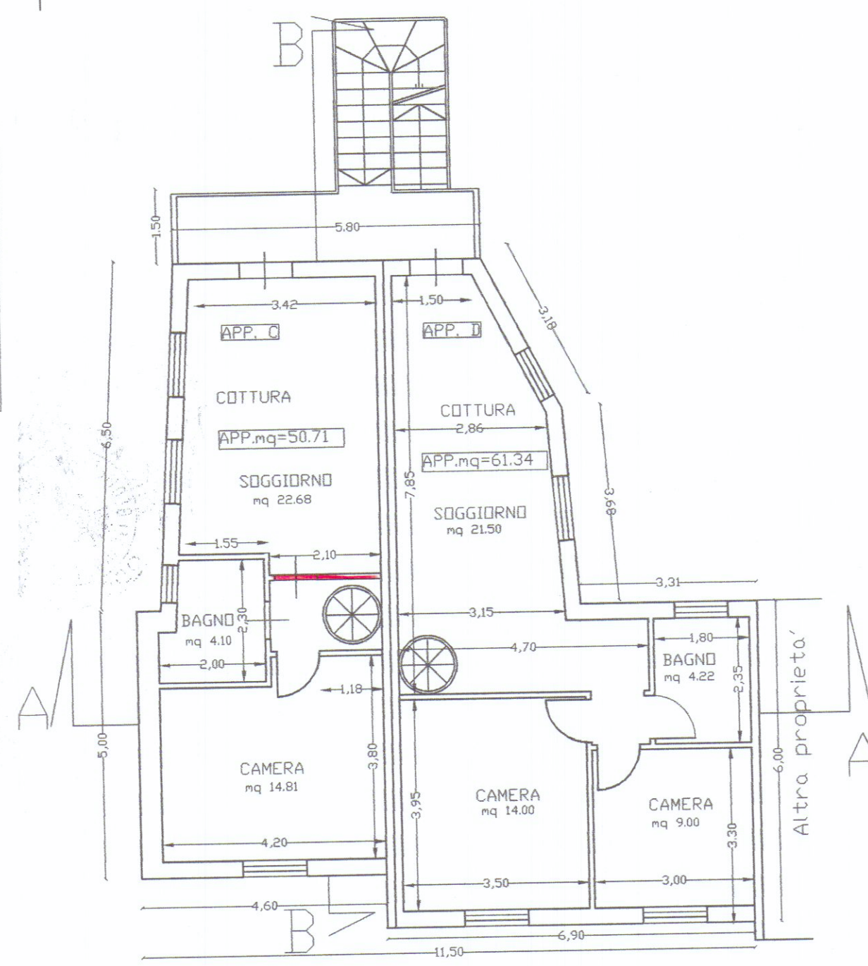
PIANO PRIMO
