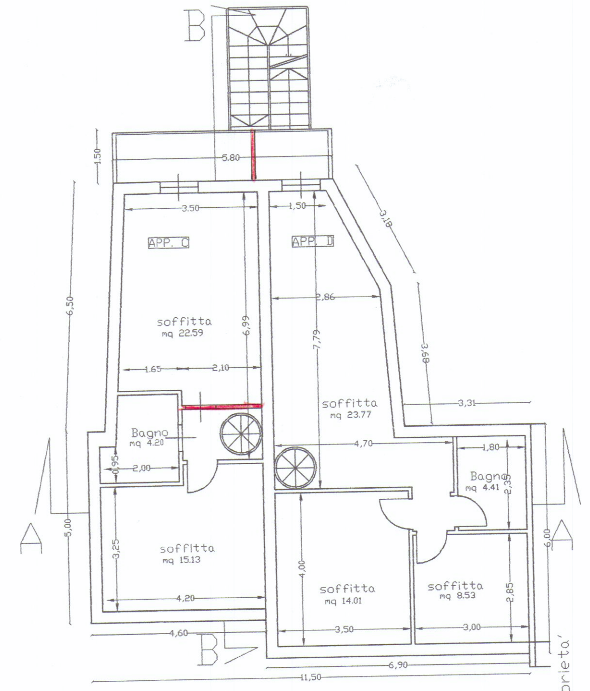
PIANO SOTTOTETTO
