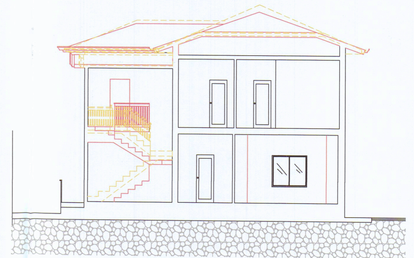
SEZIONE A-A
