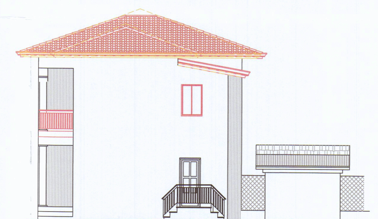
PROSPETTO EST
