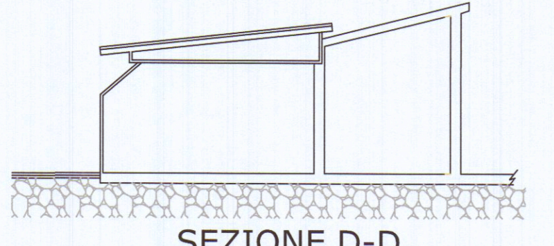
SEZIONE D-D
