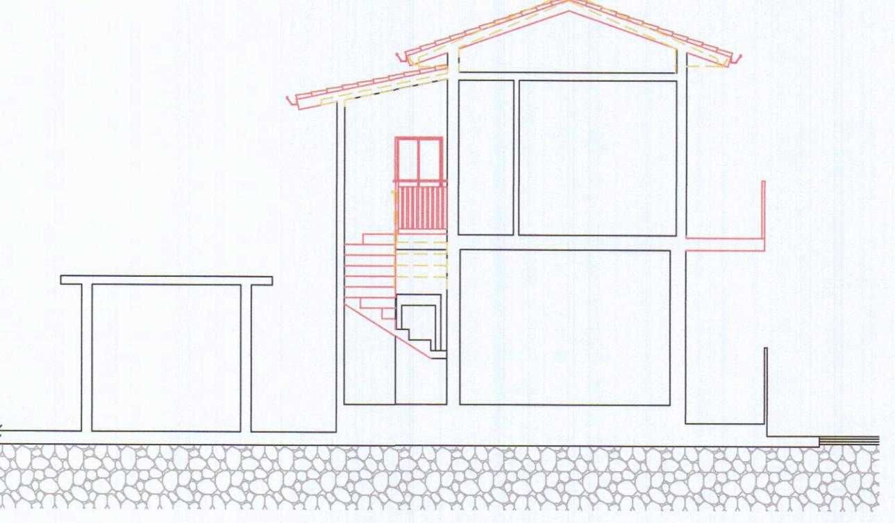
SEZIONE C-C
