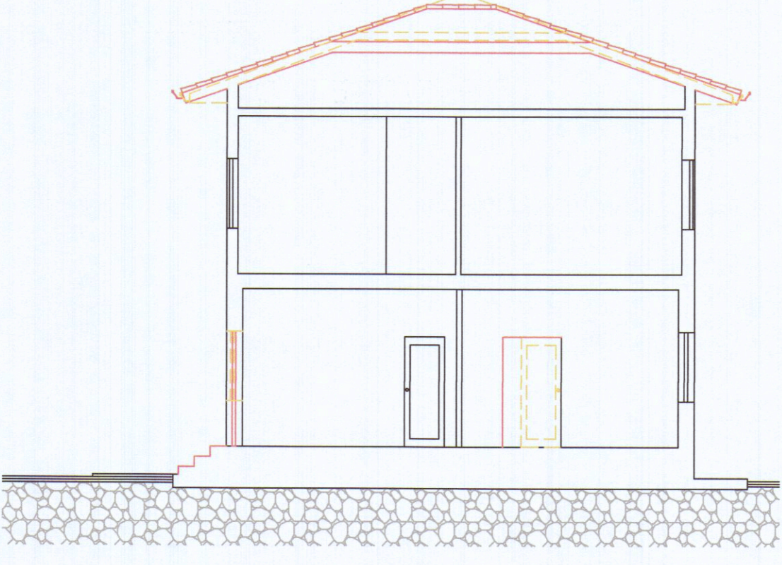
SEZIONE B-B
