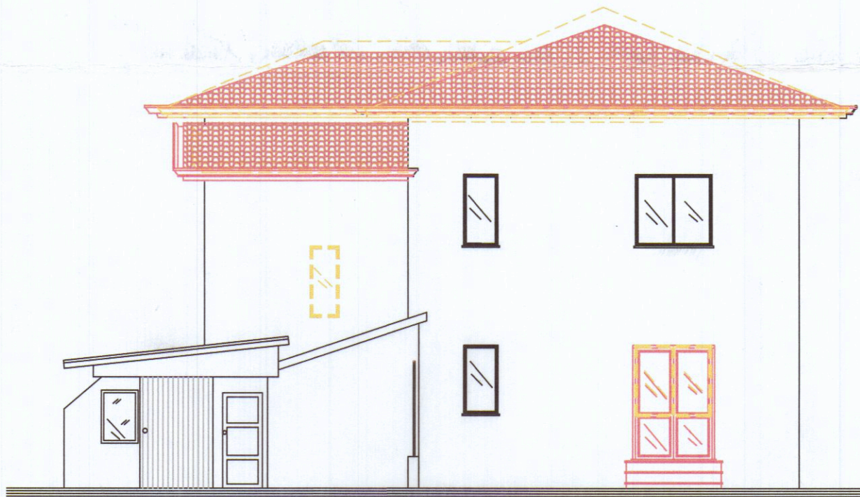
PROSPETTO NORD
