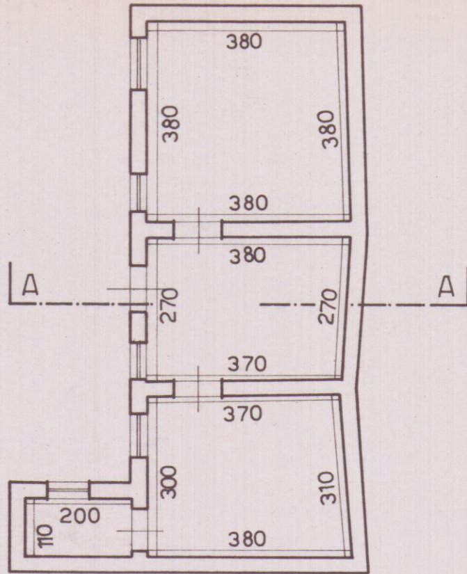
PIANTA LOCALE DI DEPOSITO
