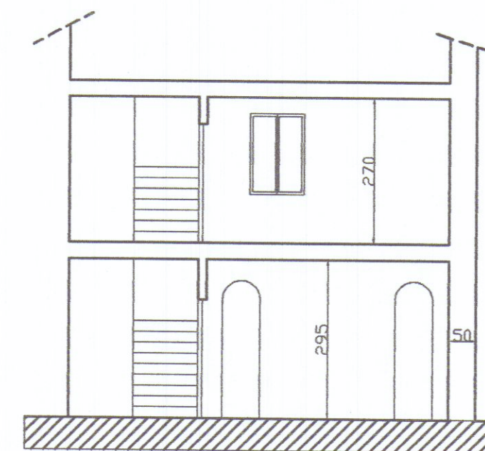
Sezione B-B
