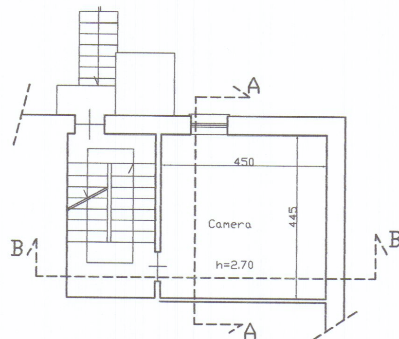
Pianta Piano Primo Cappellini
