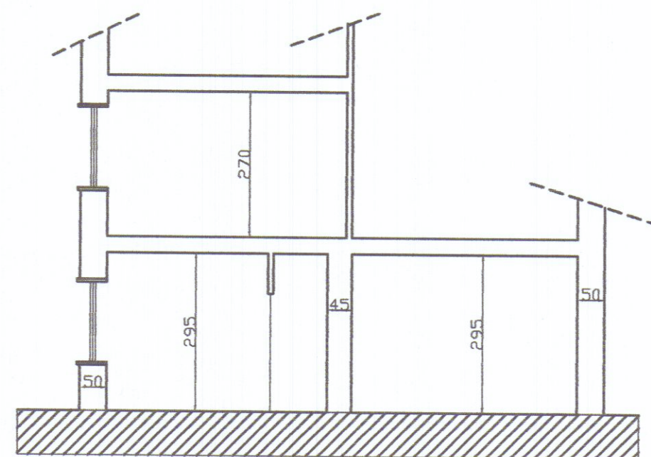
Sezione A-A
