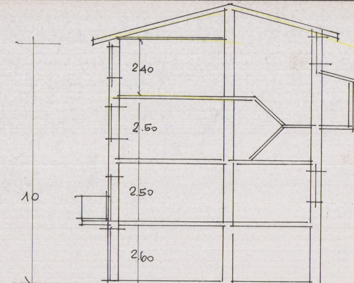
SEZIONE ESISTENTE
