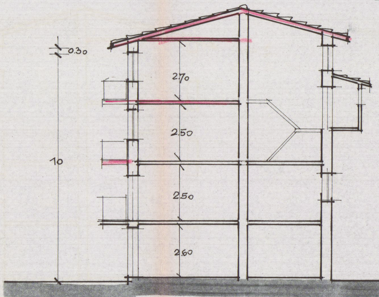
SEZIONE
