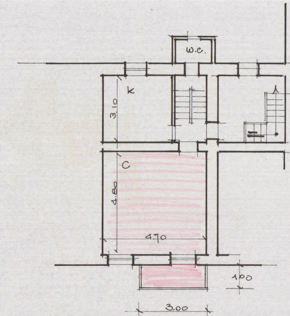
PIANTA P. 2°-3°
