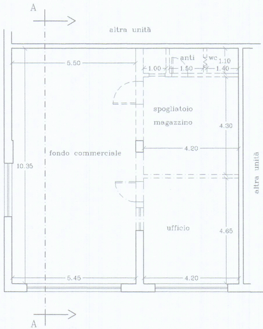
PIANTA
