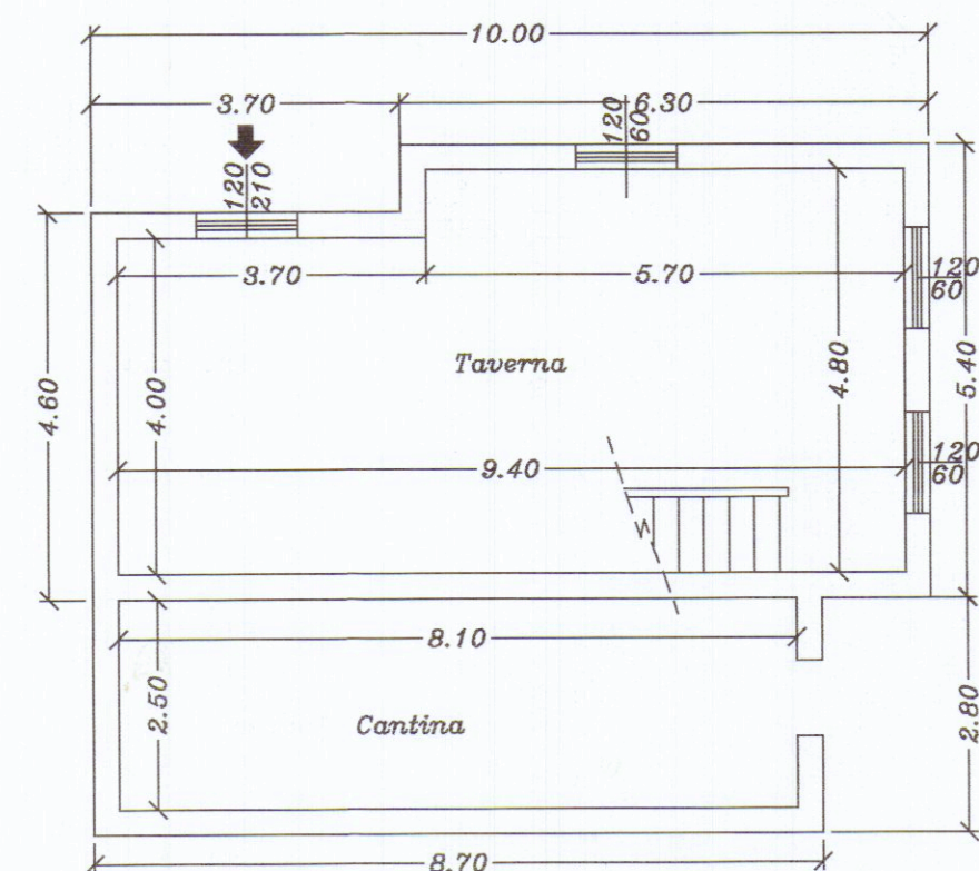
Pianta piano Interrato
