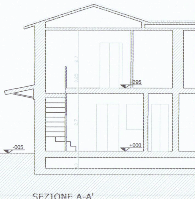
SEZIONE A-A' scala 1.100
