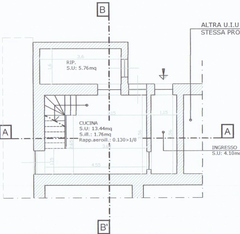
PIANTA PIANO TERRA scala 1.100
