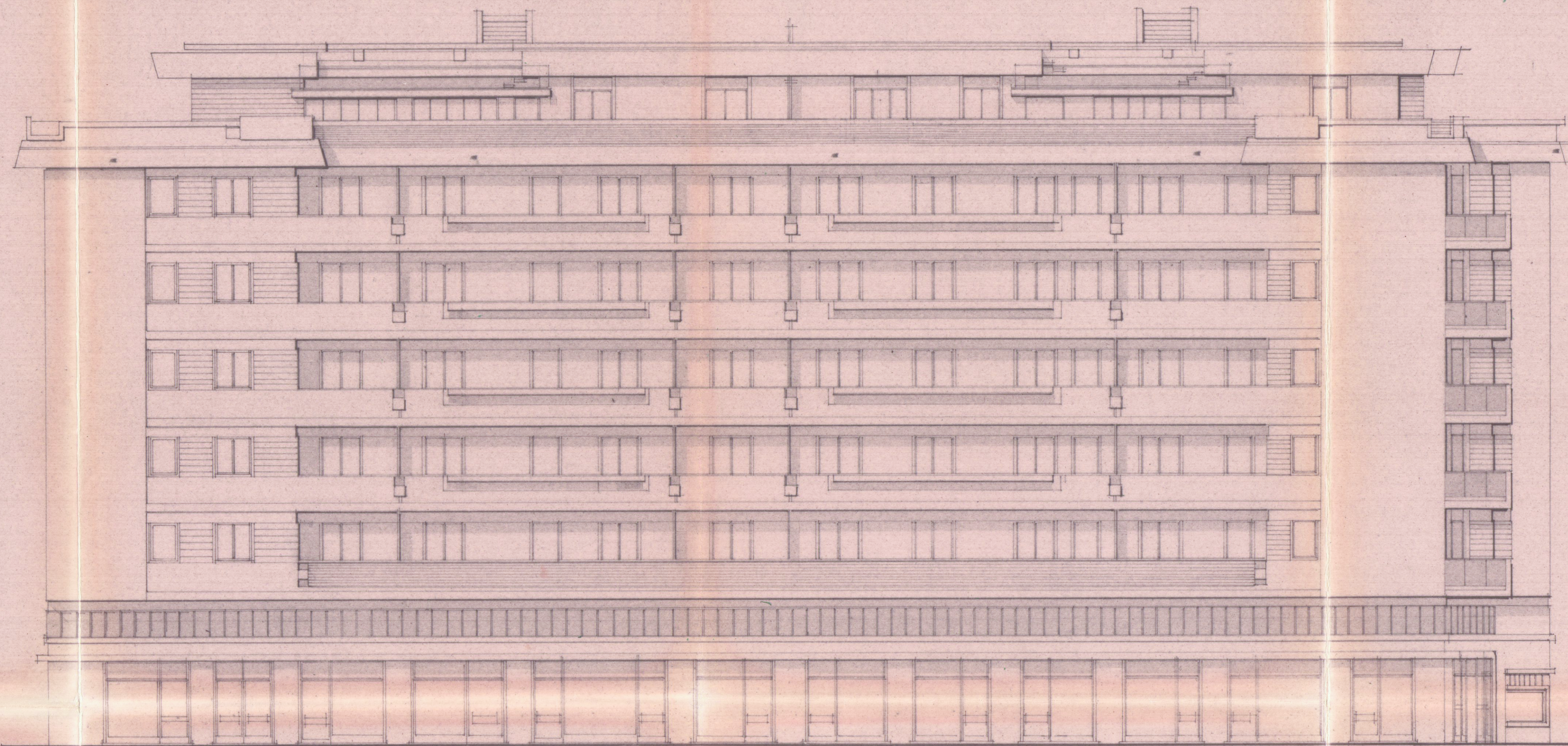
PROSPETTO NORD
