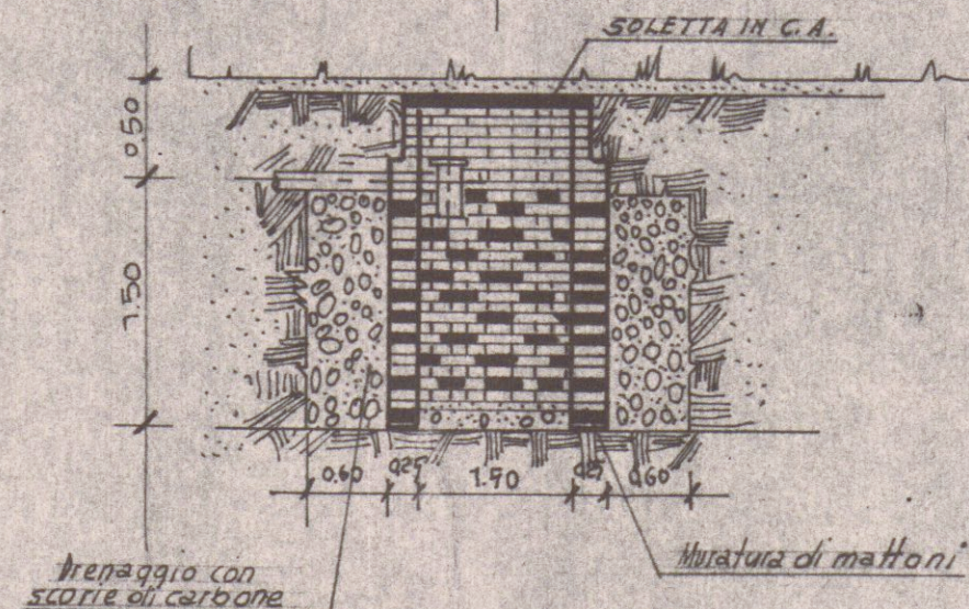
SEZIONE A-B
