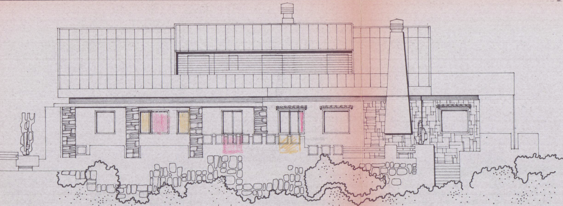
PROSPETTO PRINCIPALE SUD CON MODIFICHE
