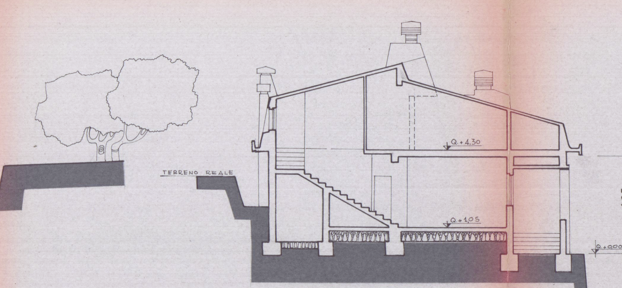
SEZIONE TRASVERSALE A-B
