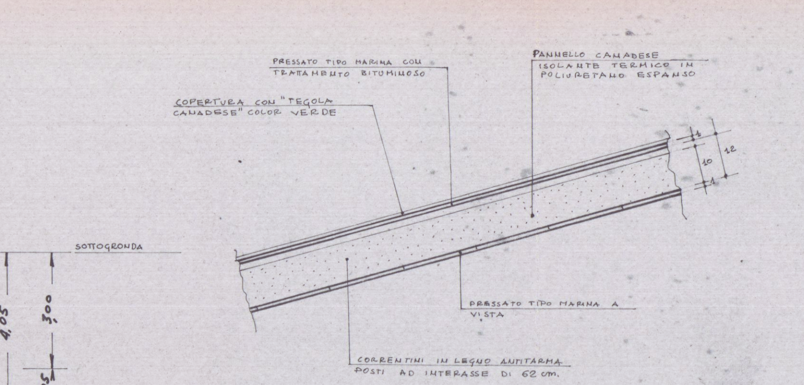
PARTICOLARE COSTRUTTIVO DEL TETTO - RAPP. 1/10
