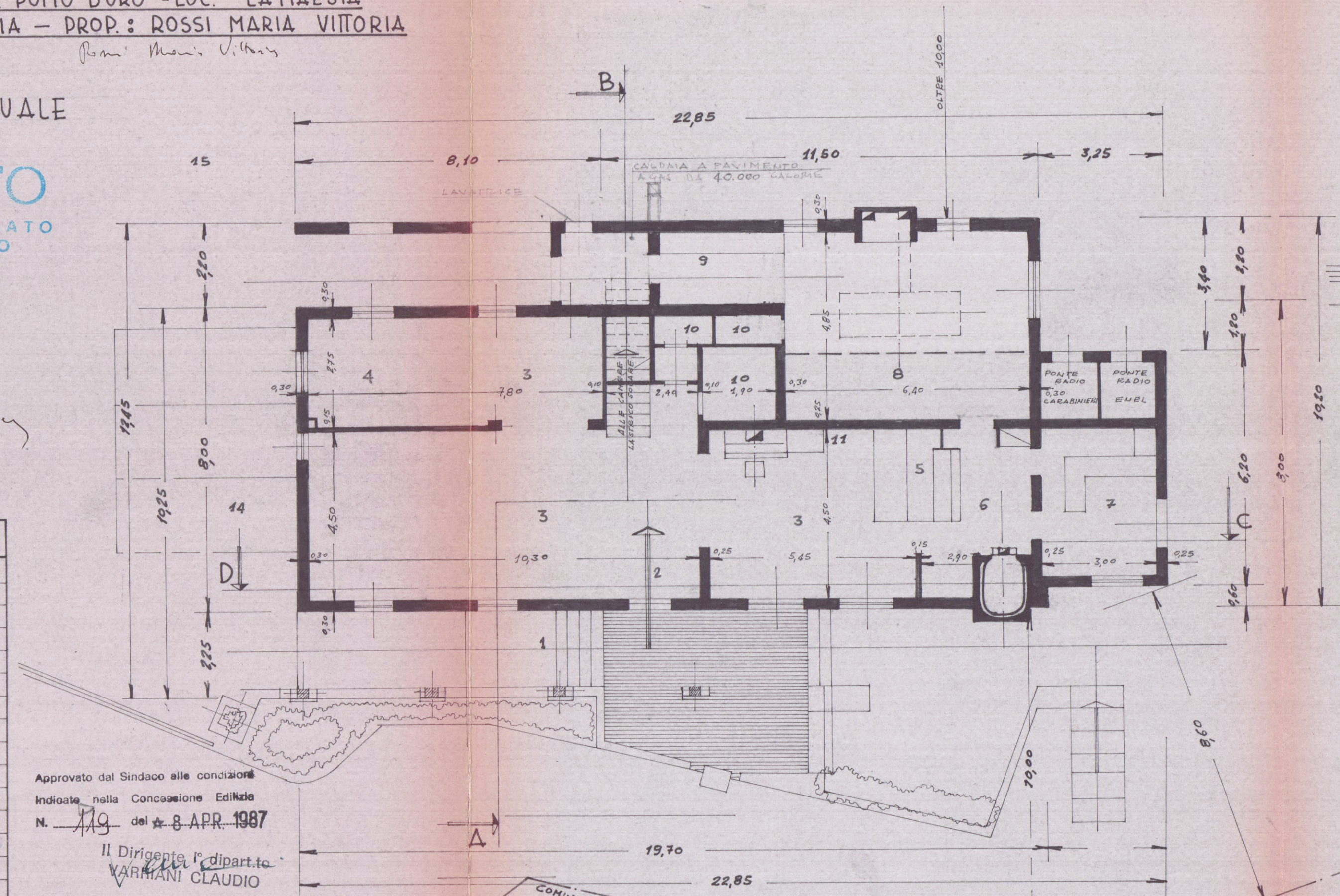
PIANTA PIANO RIALZATO CON
