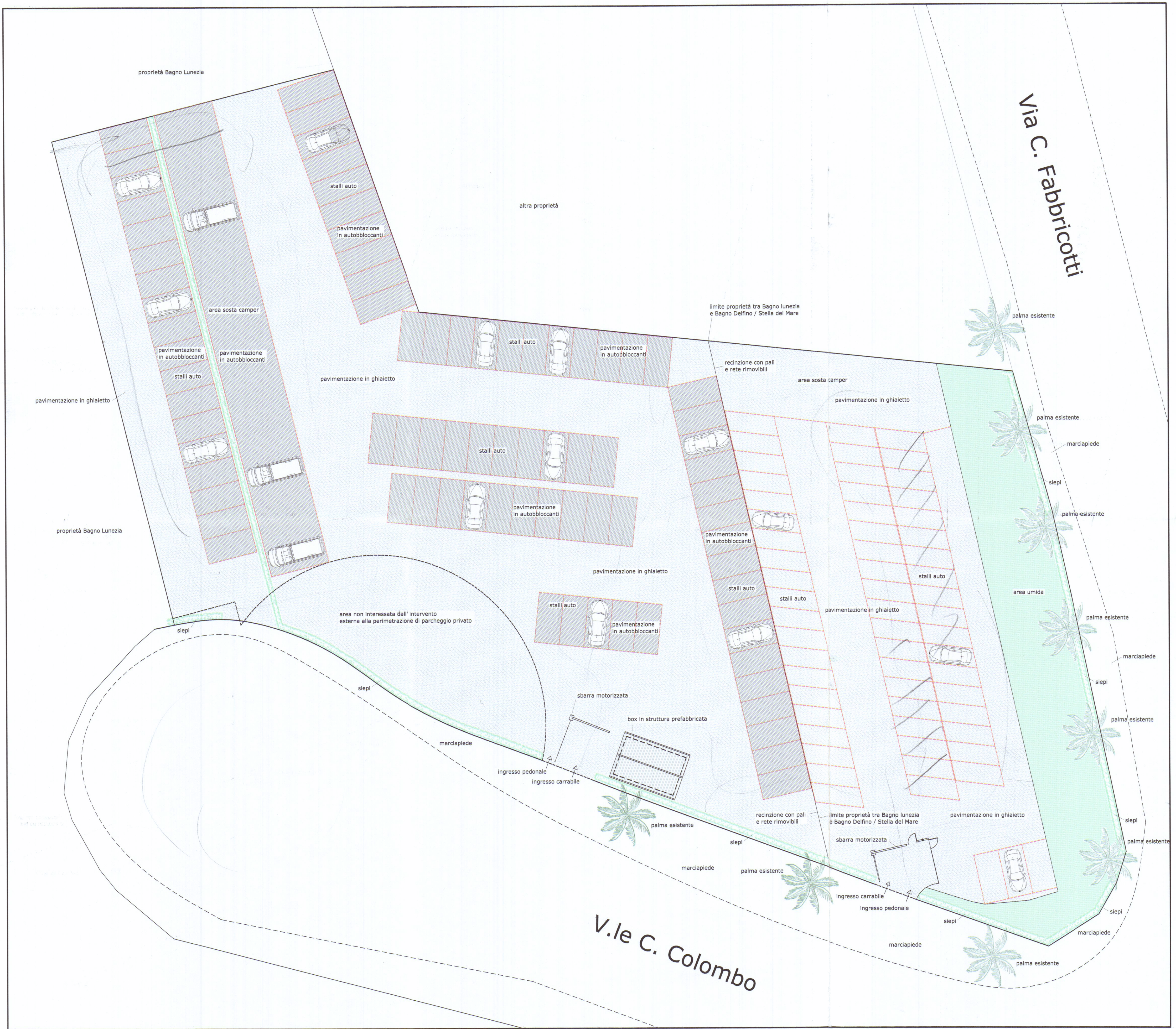
PLANIMETRIA DETTAGLIATA scala 1:200
