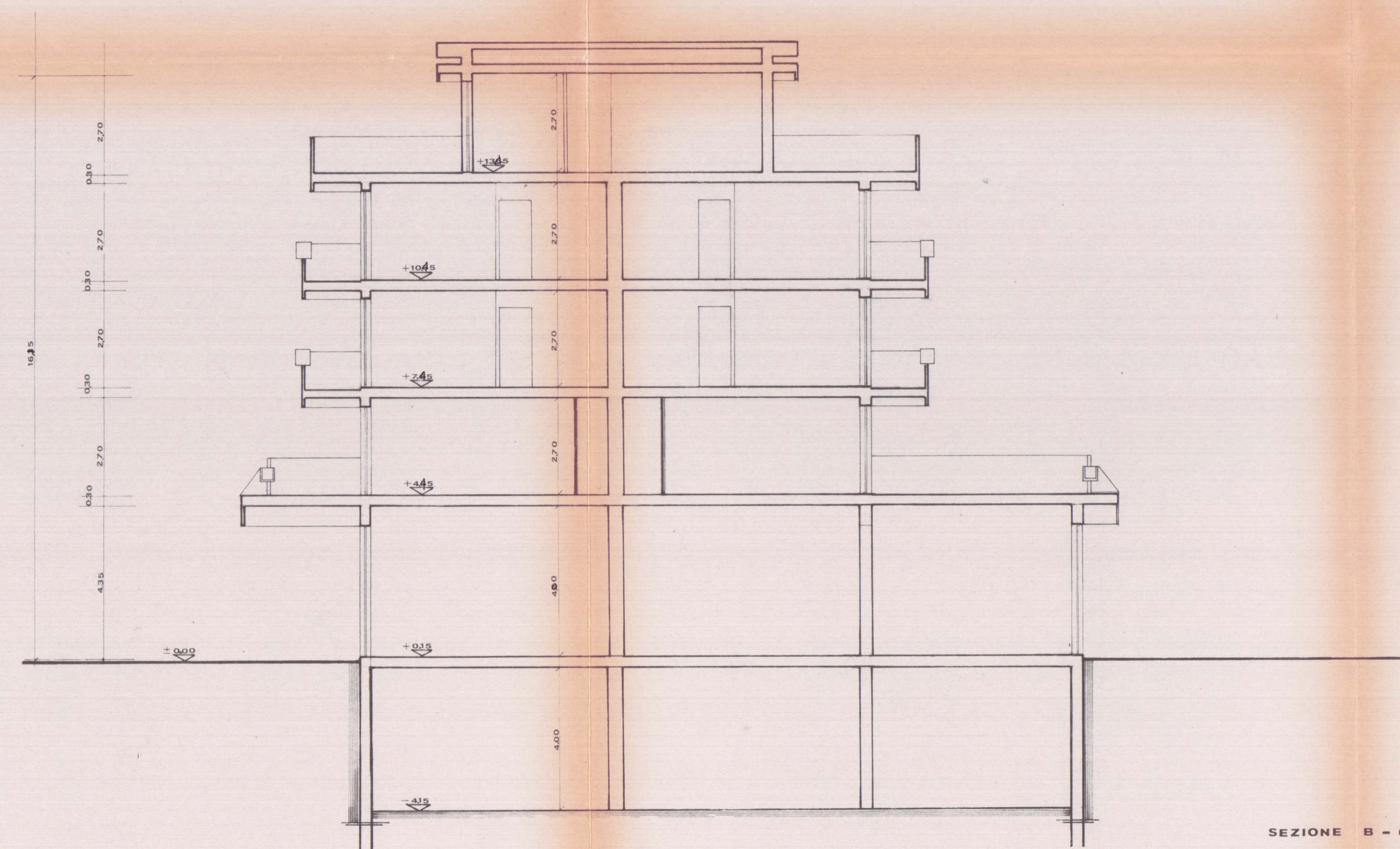
SEZIONE B - B
