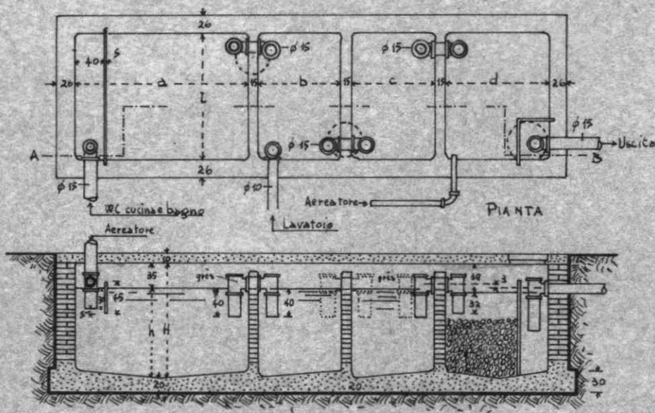
SEZIONE A-B
