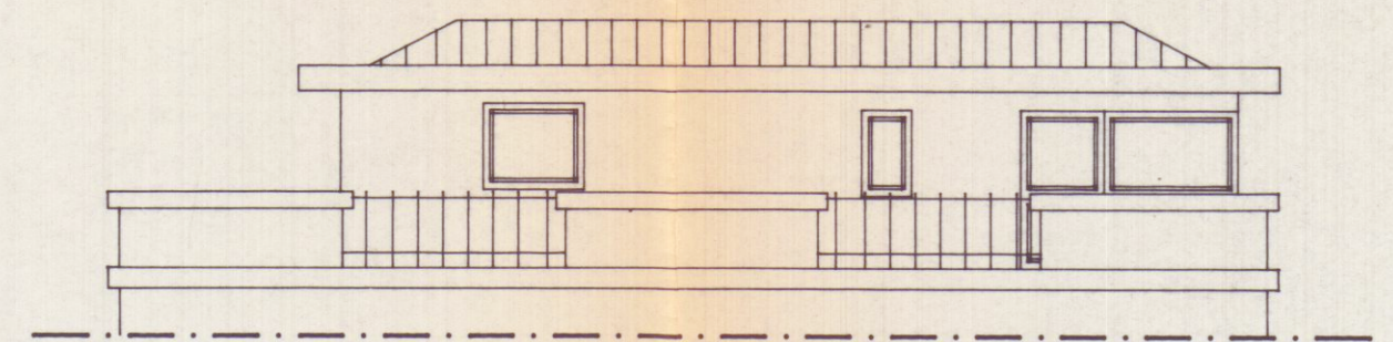
Prospetto Ovest
