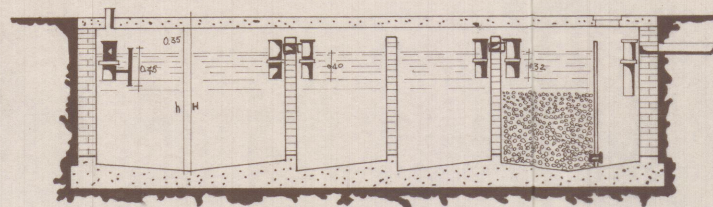
SEZIONE A-B
