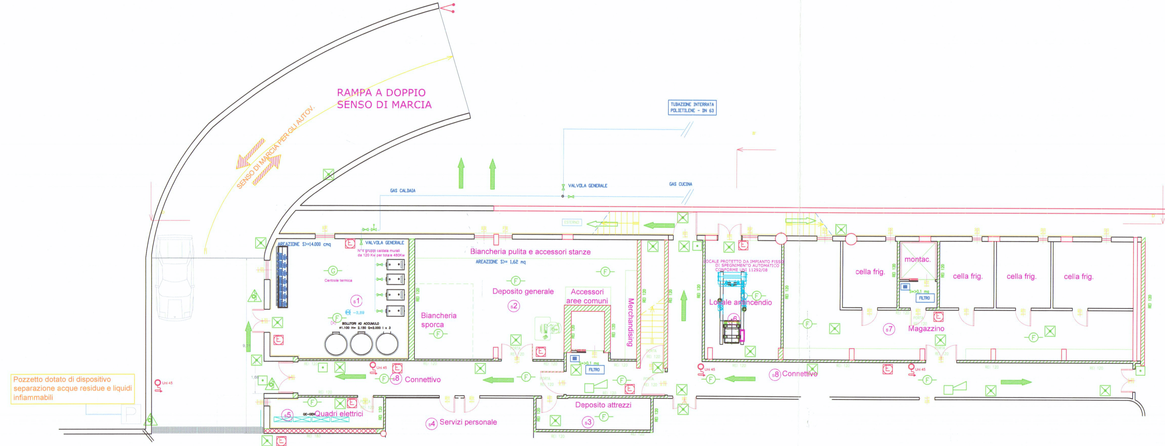
PIANTA SCALA 1:100 LOCALI TECNICI
