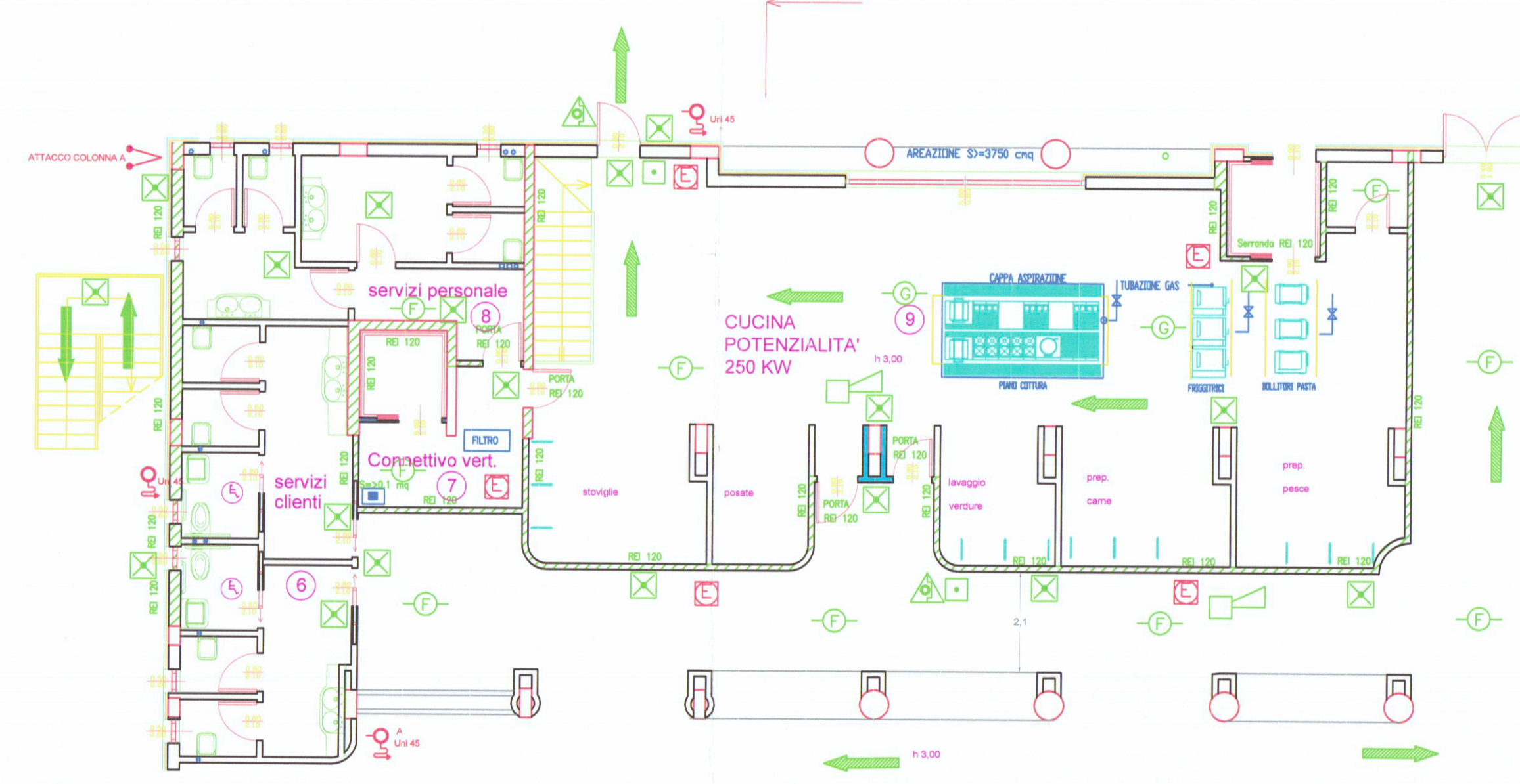
PIANTA SCALA 1:100 LOCALE CUCINA
