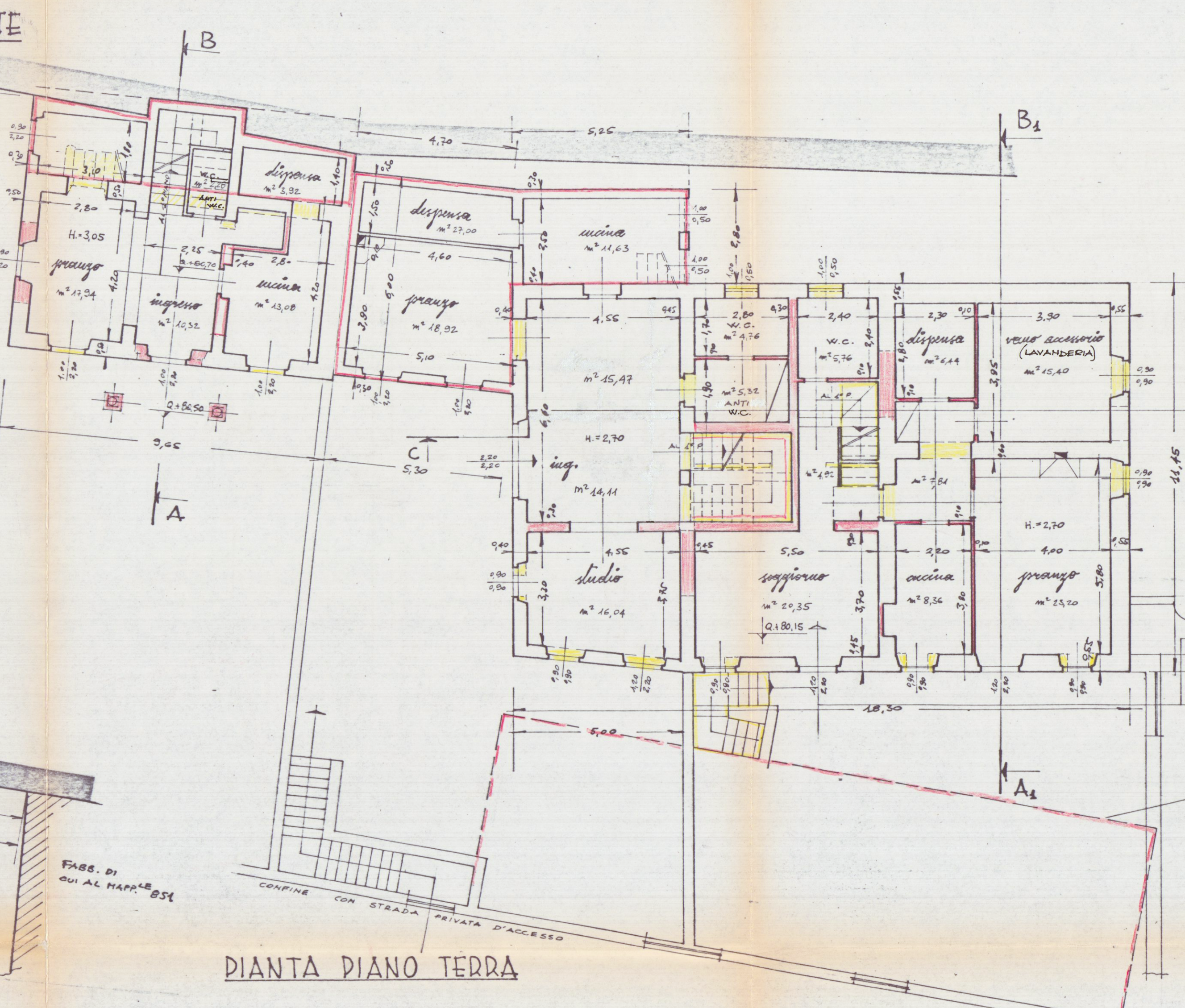
PIANTA GARAGE INTERRATO
