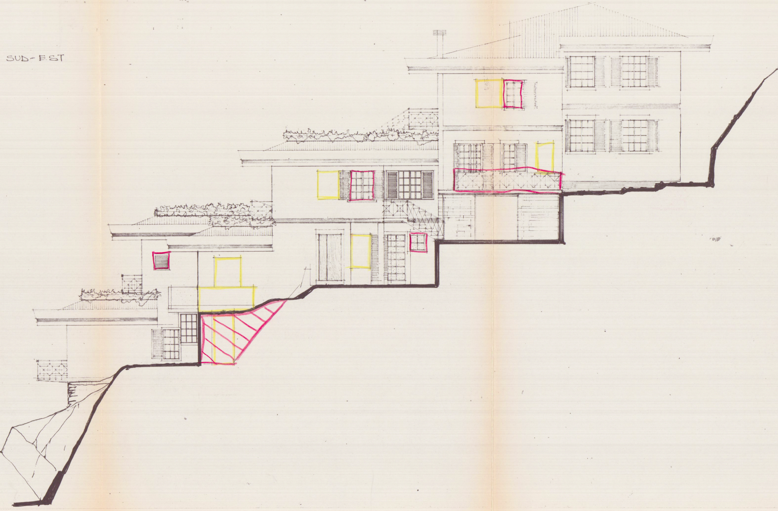
PROSPETTO OVEST SEZIONE BB' TAV. 9
