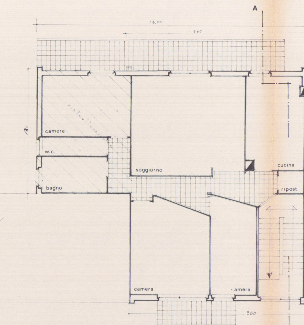
1° PIANO
