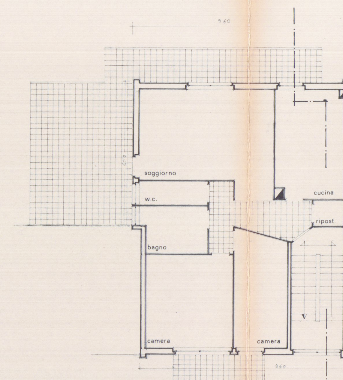
2° PIANO
