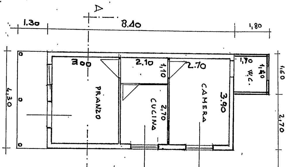
PIANTA
