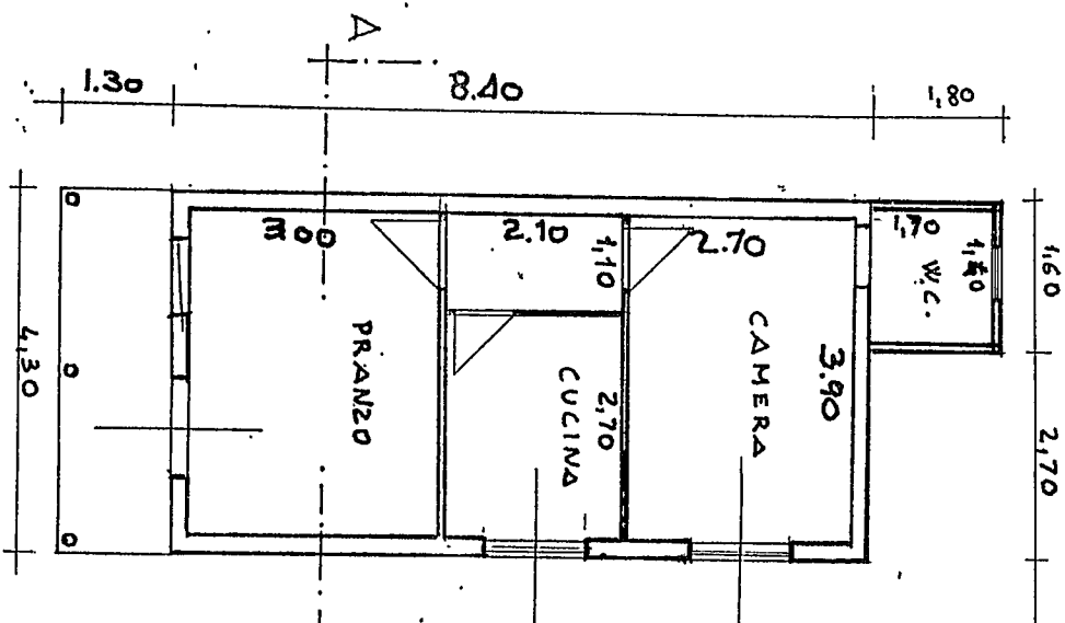
PIANTA
