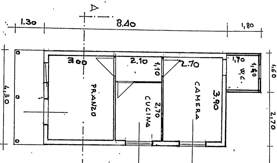
PIANTA
