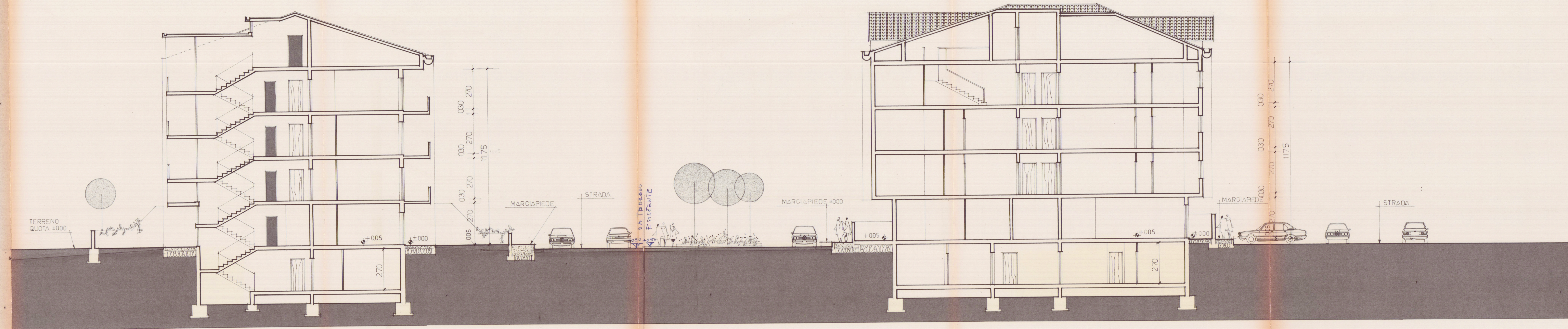
sezione a:a
