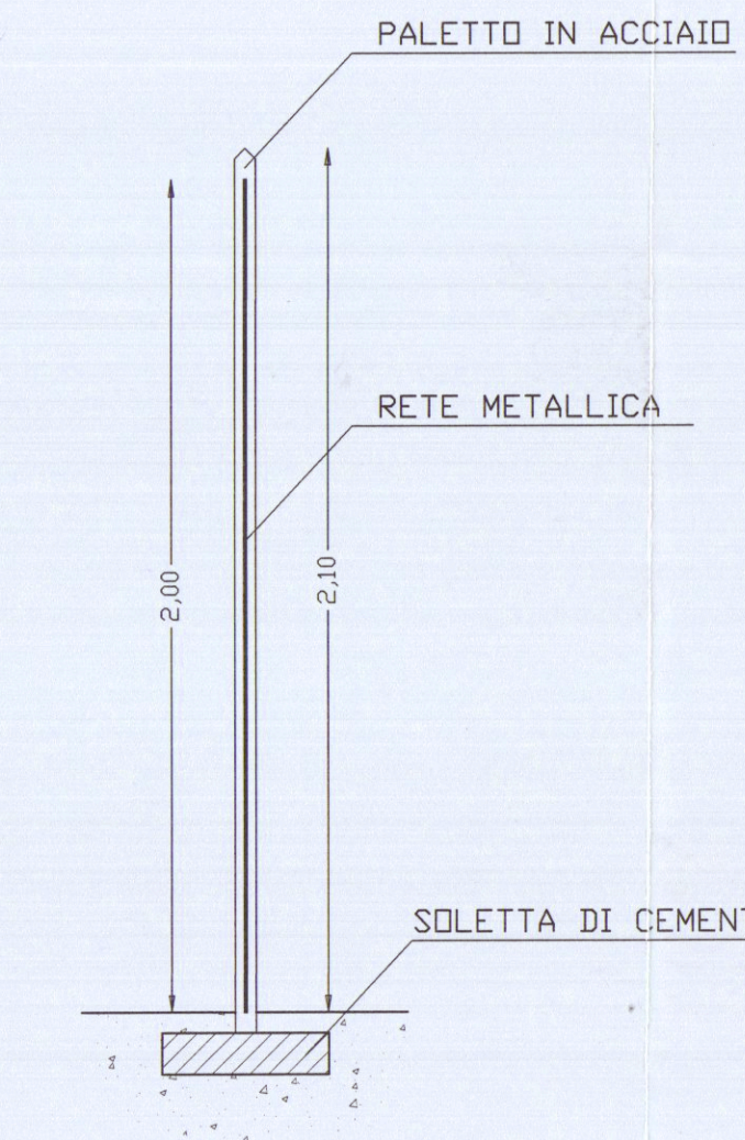
SEZIONE A-A (Rapp.Scala 1/20)
