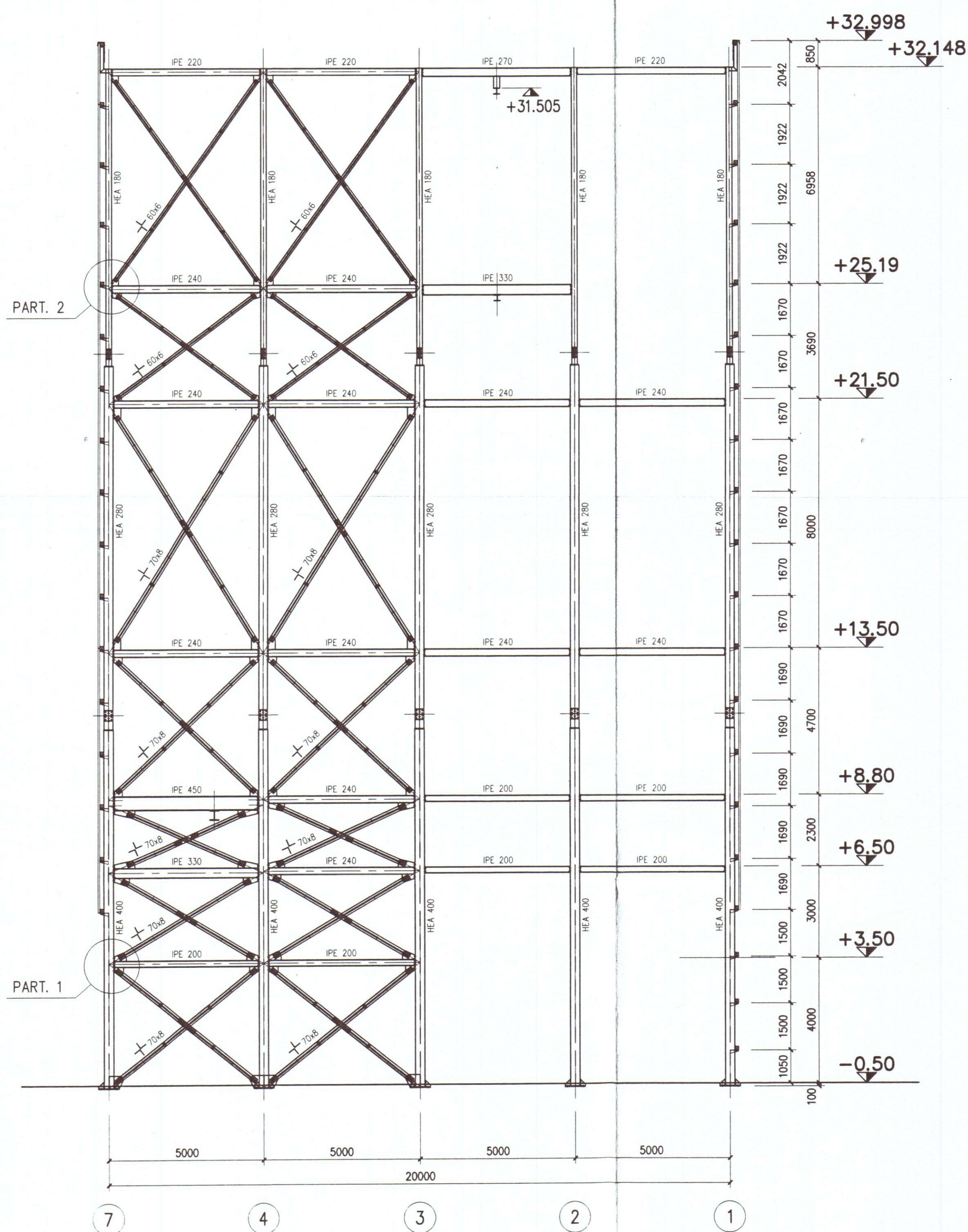
ALLINEAMENTO A scala 1:100
