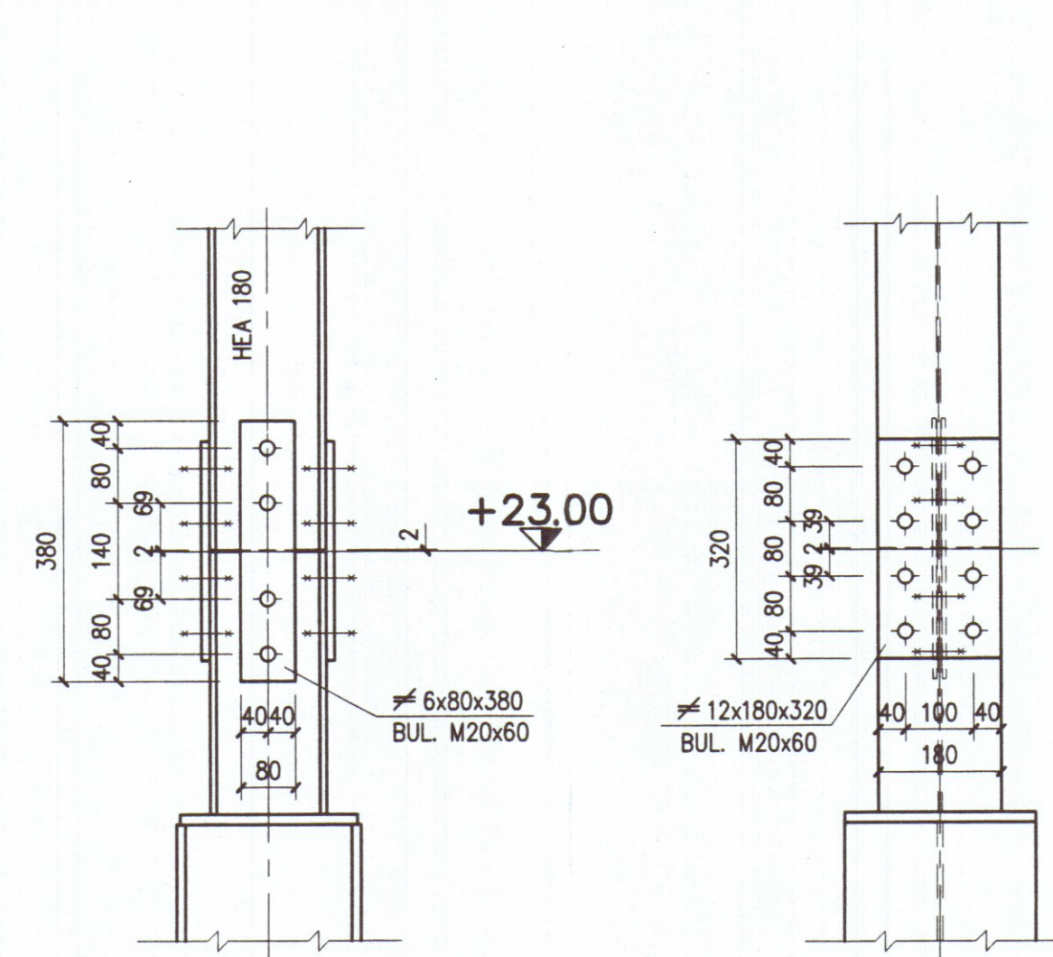
PART. GIUNTO COLONNE HEA 180
