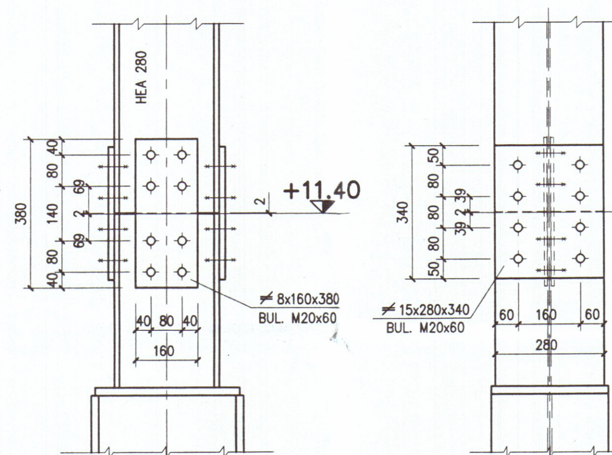
PART. GIUNTO COLONNE HEA 280
