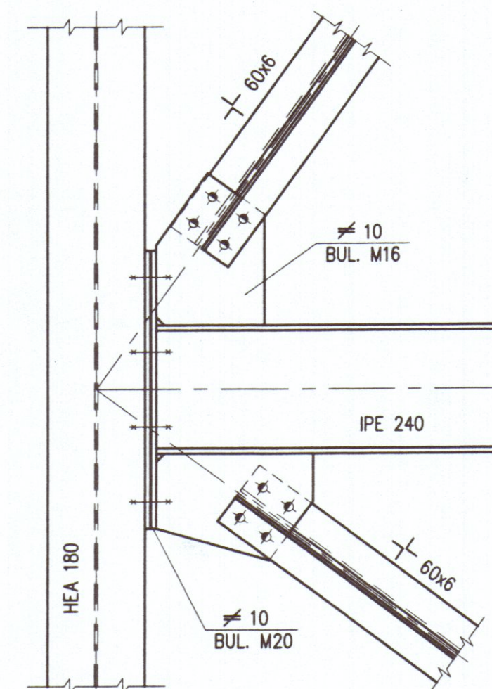
PART. 2 scala 1:10
