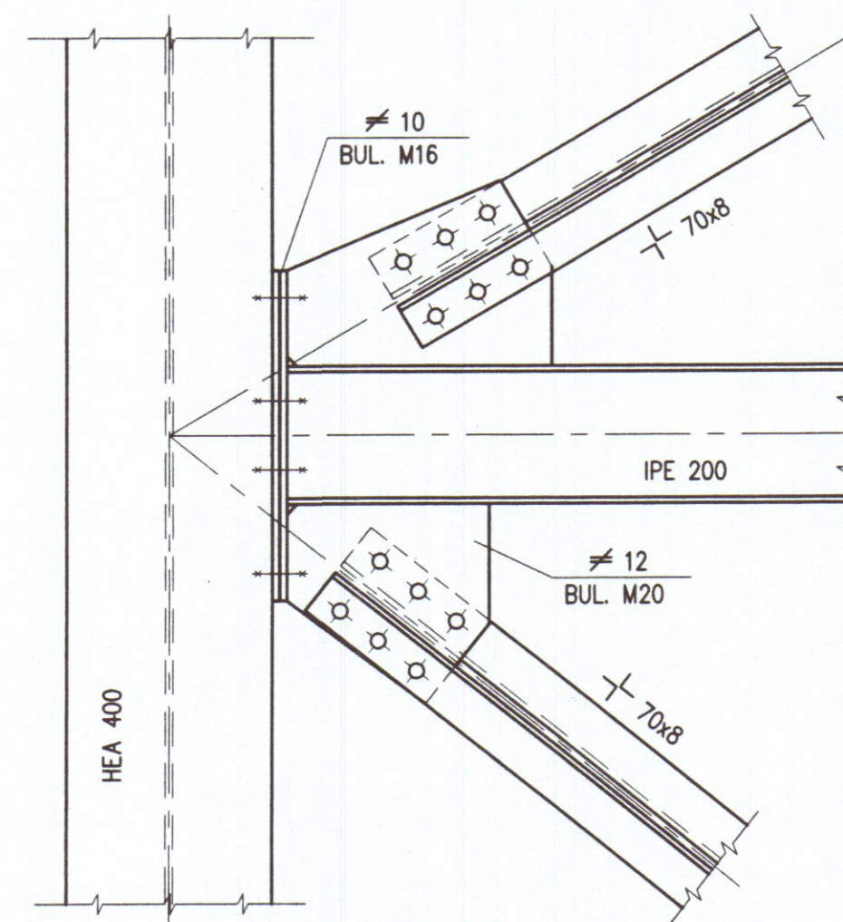
PART. 1 scala 1:10
