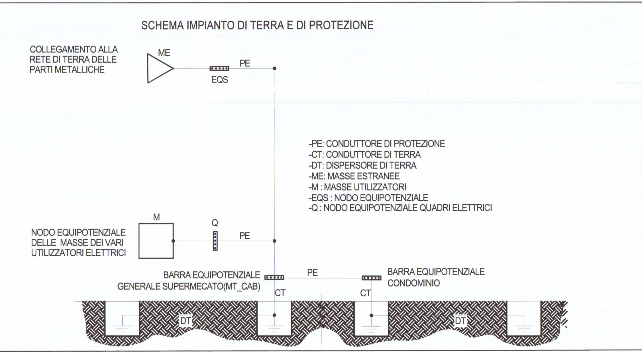
Schema impianto di terra generale
