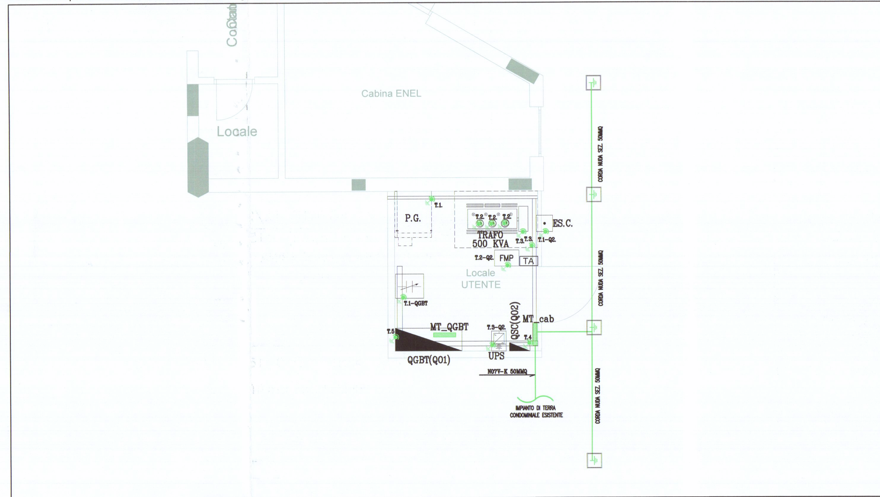
Planimetria impianto di terra locale tecnico e collettore generale scala 1:50
