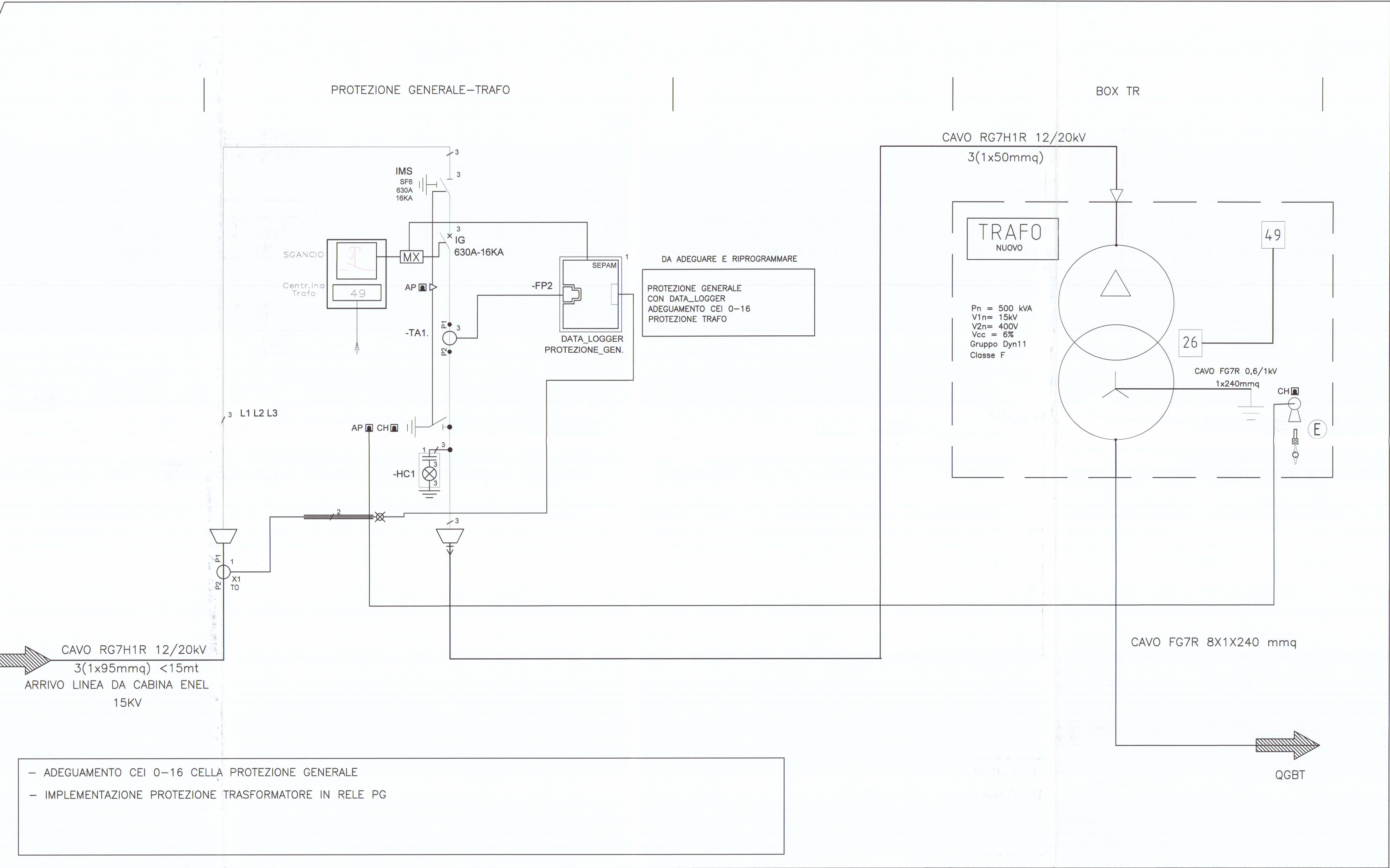
schema unifilare MT/BT
