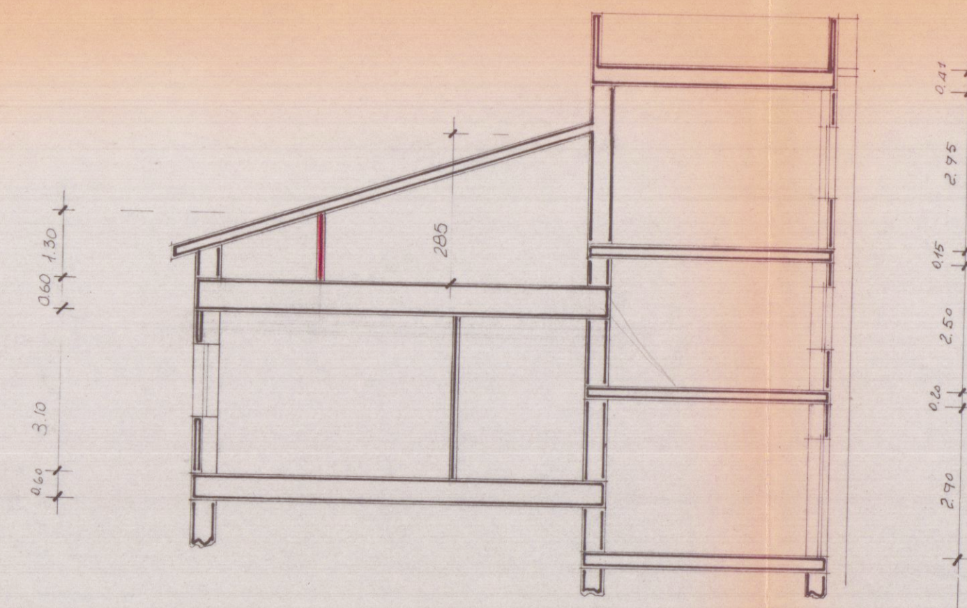
sezione A-A'
