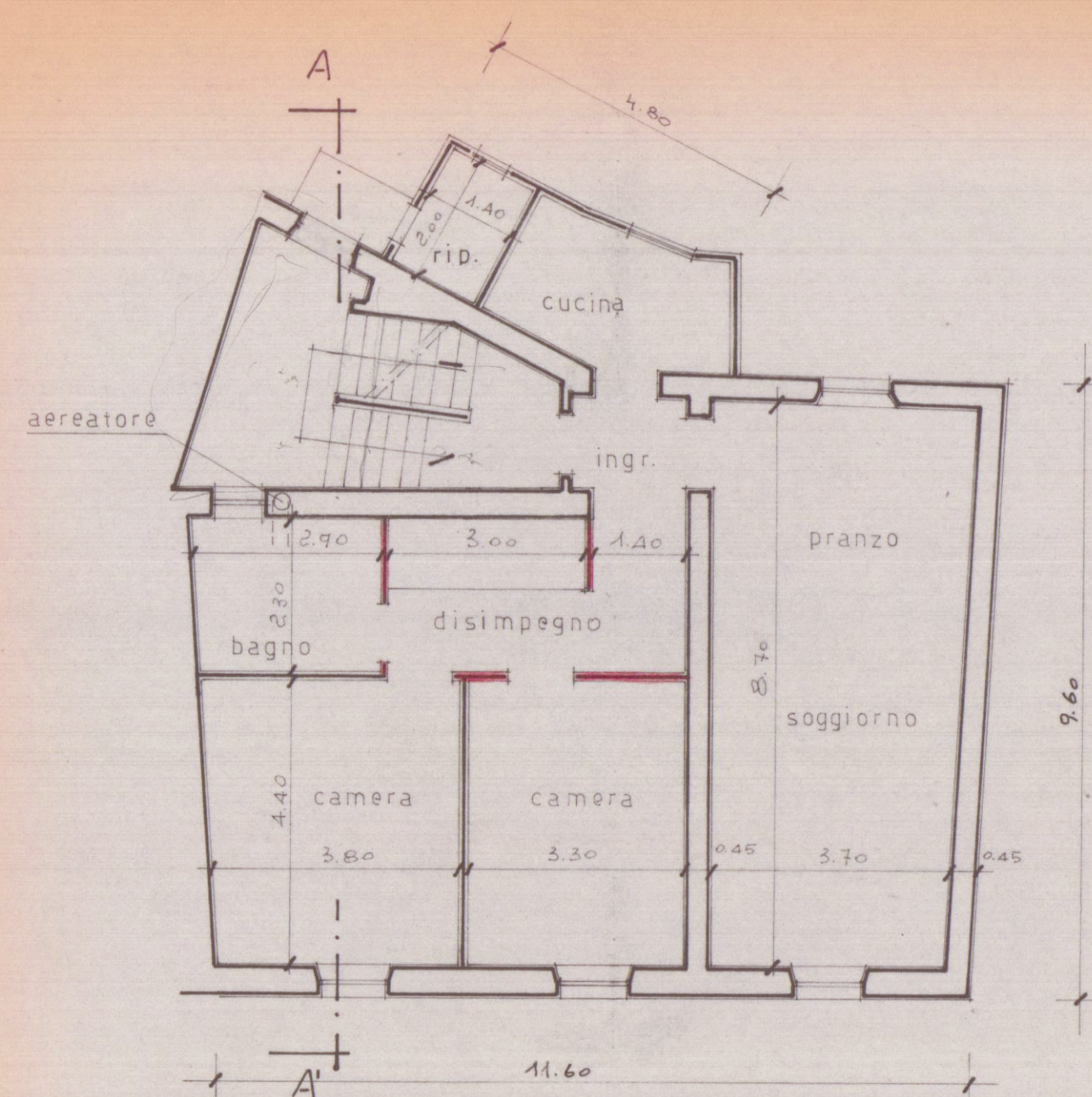
piano terzo
