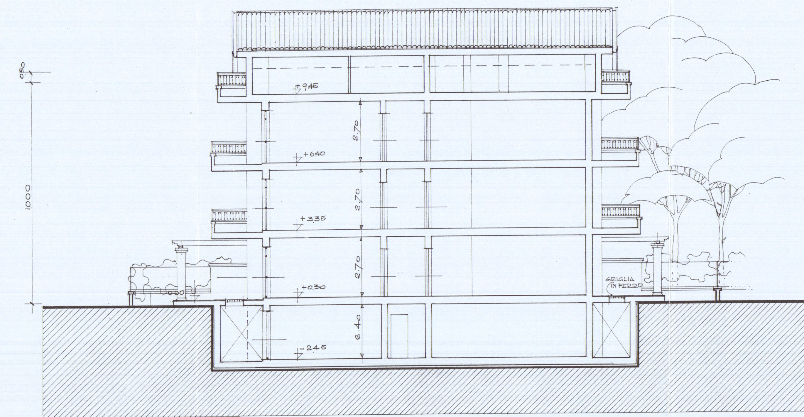
SEZIONE B-B
