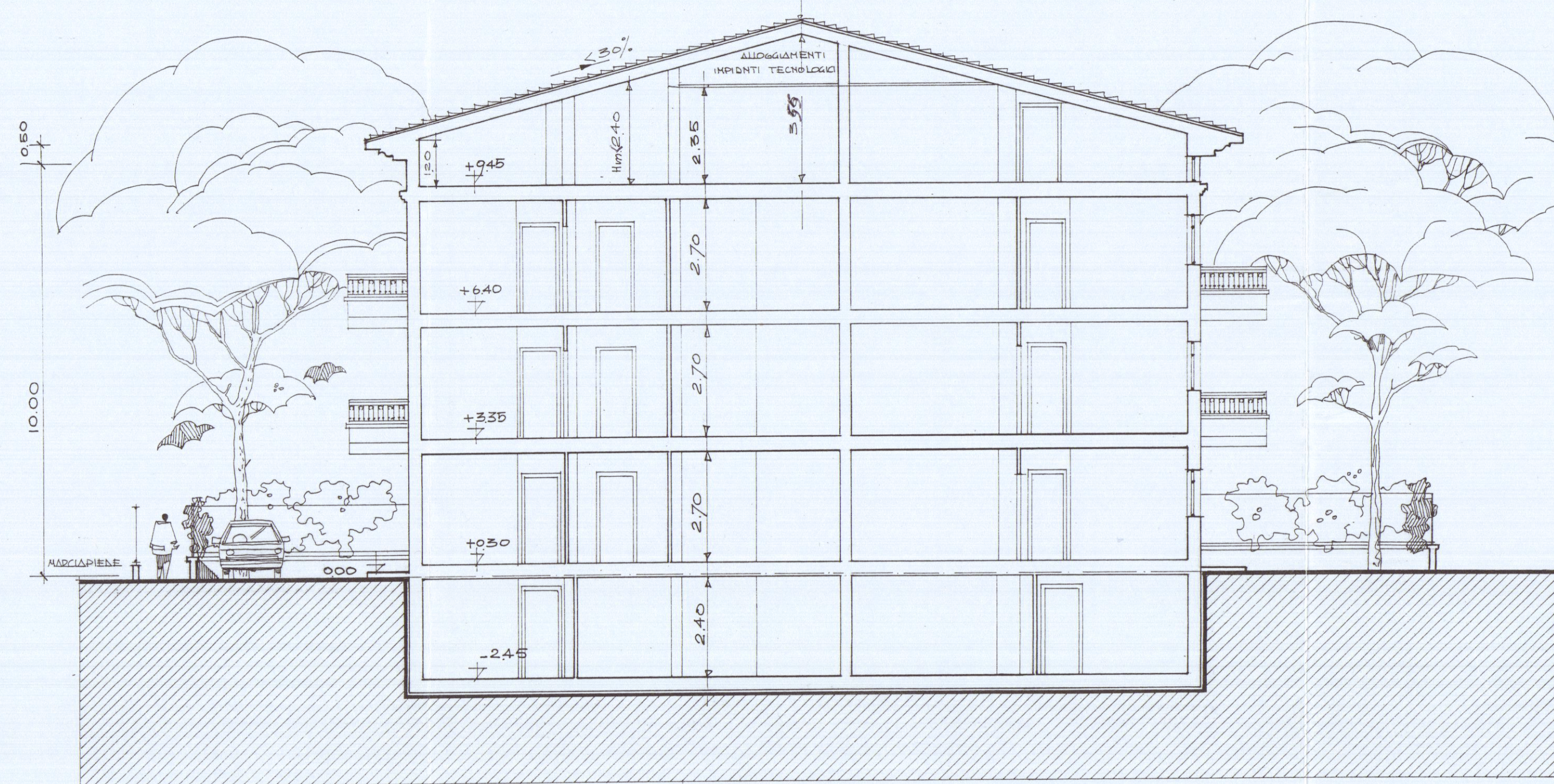
SEZIONE A-A
