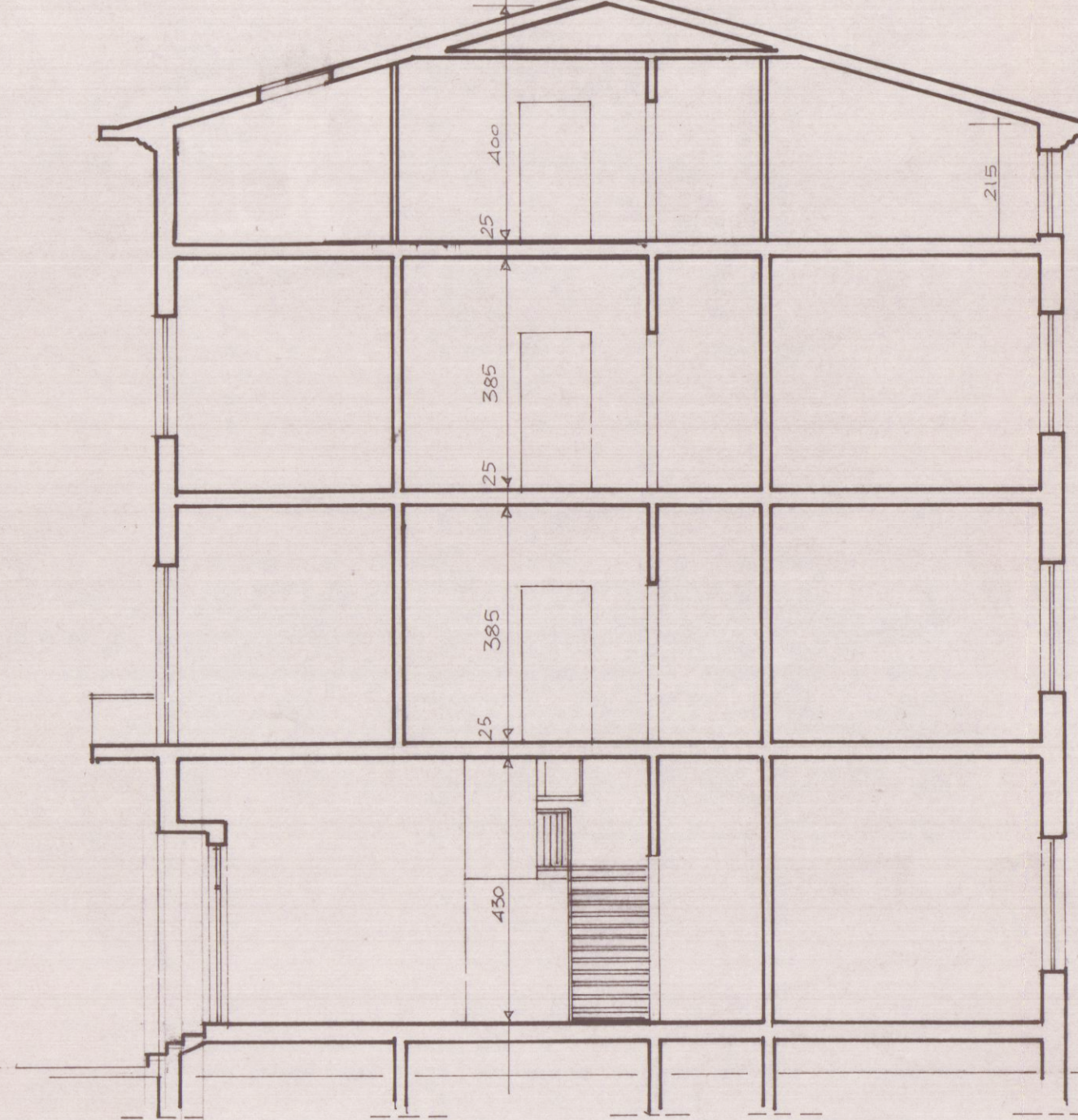
SEZIONE B-B'
