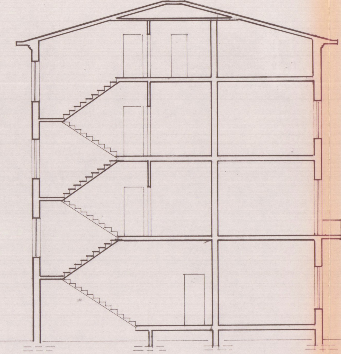
SEZIONE A-A'
