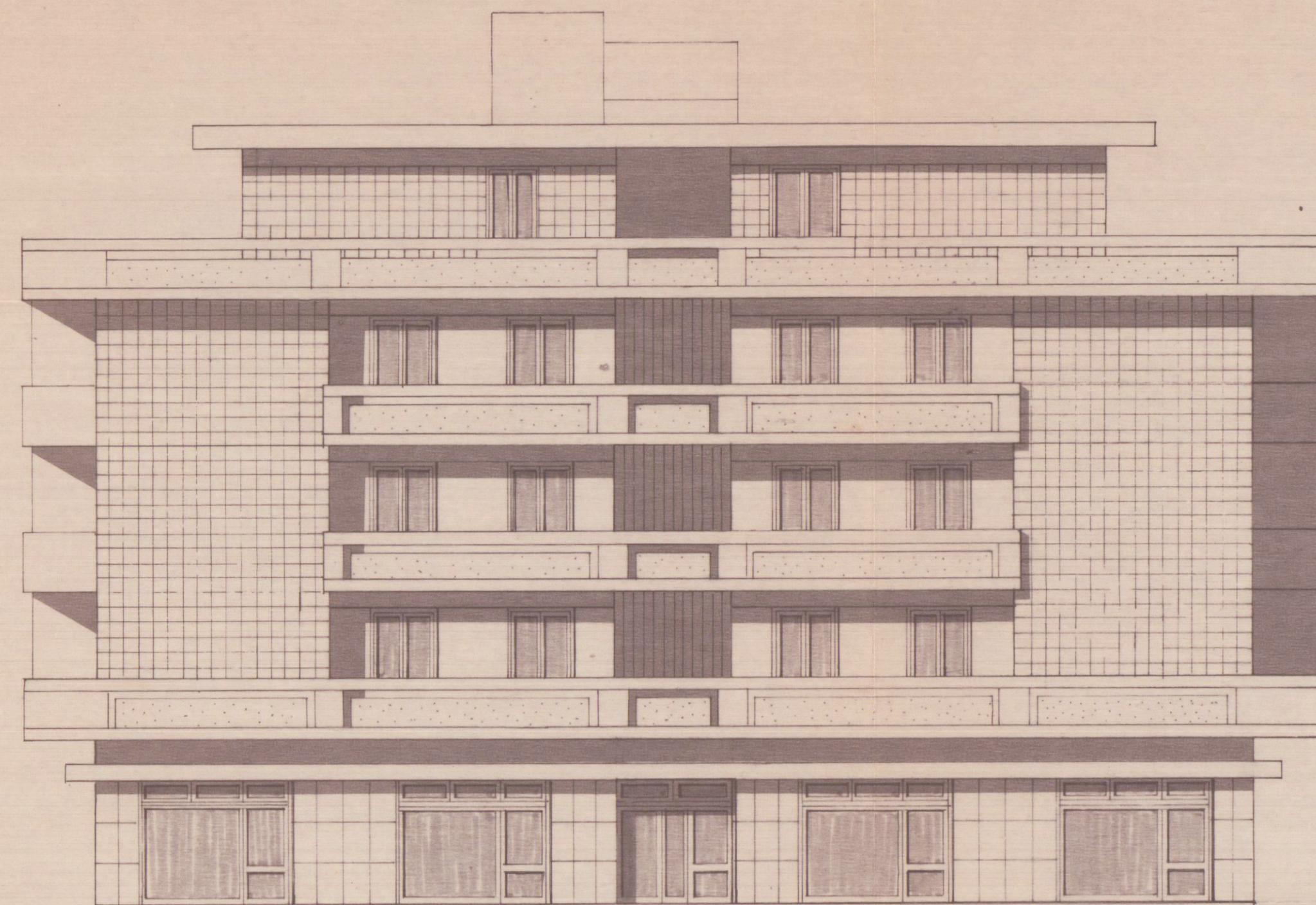
PROSPETTO NORD
