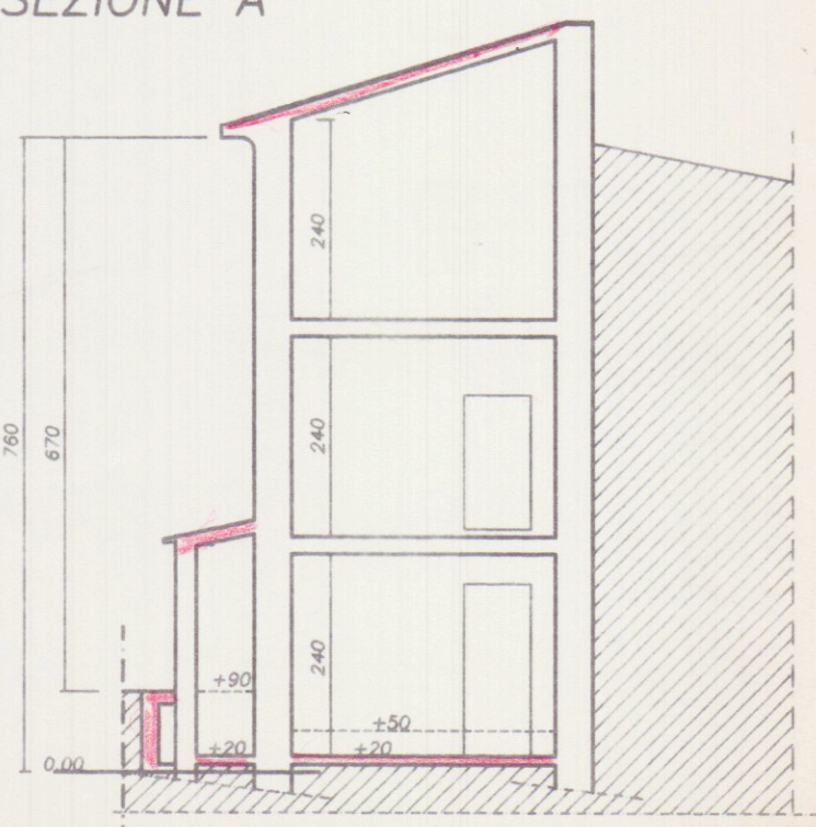
SEZIONE A
