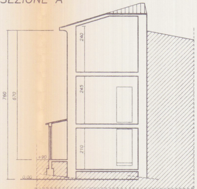
SEZIONE A
