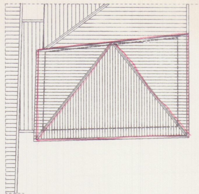
PIANTA COPERTURA
