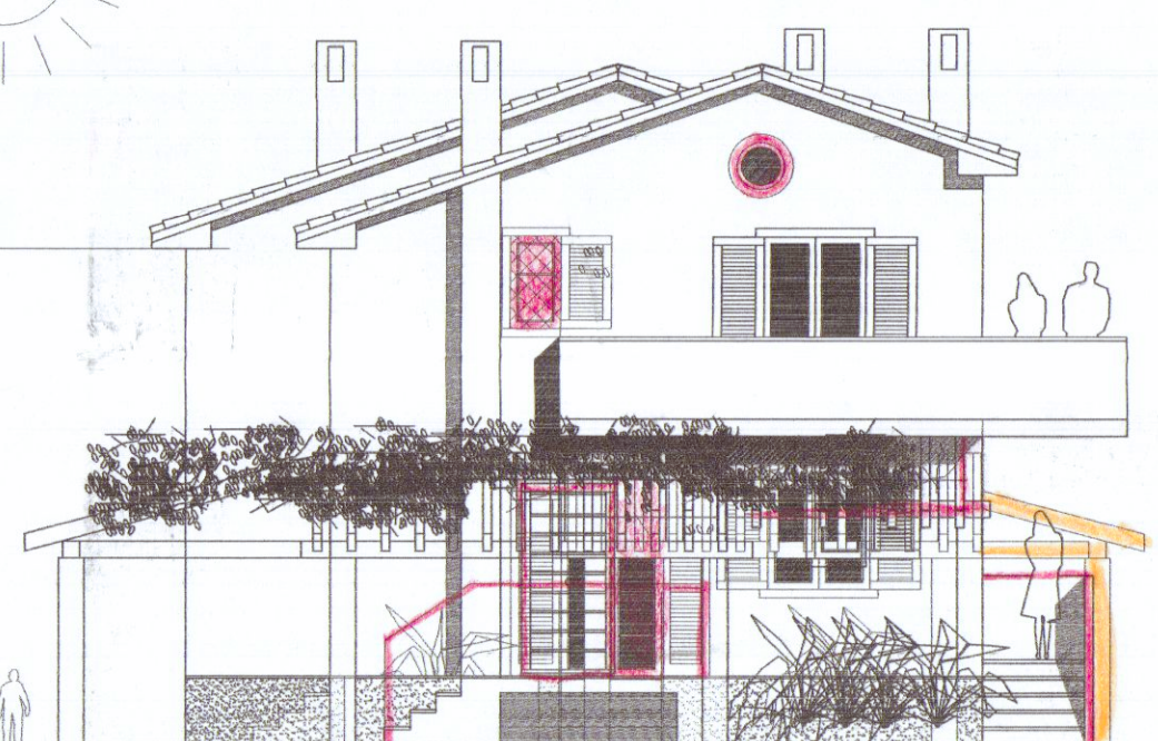
prospetto est sovrapposto
