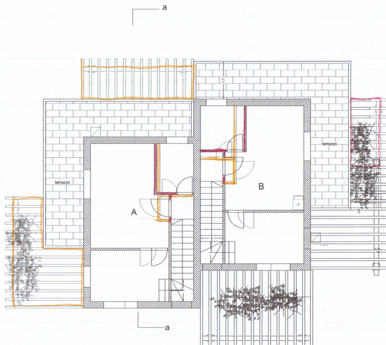
pianta piano sovrapposto
