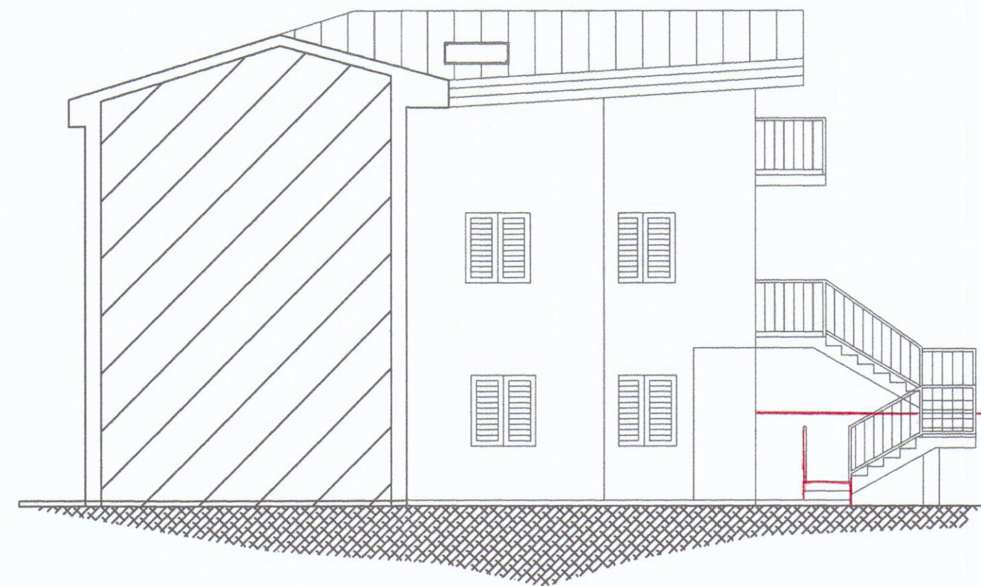
PROSPETTO OVEST
