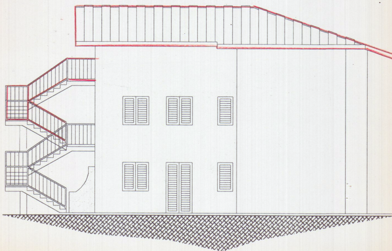
PROSPETTO EST
