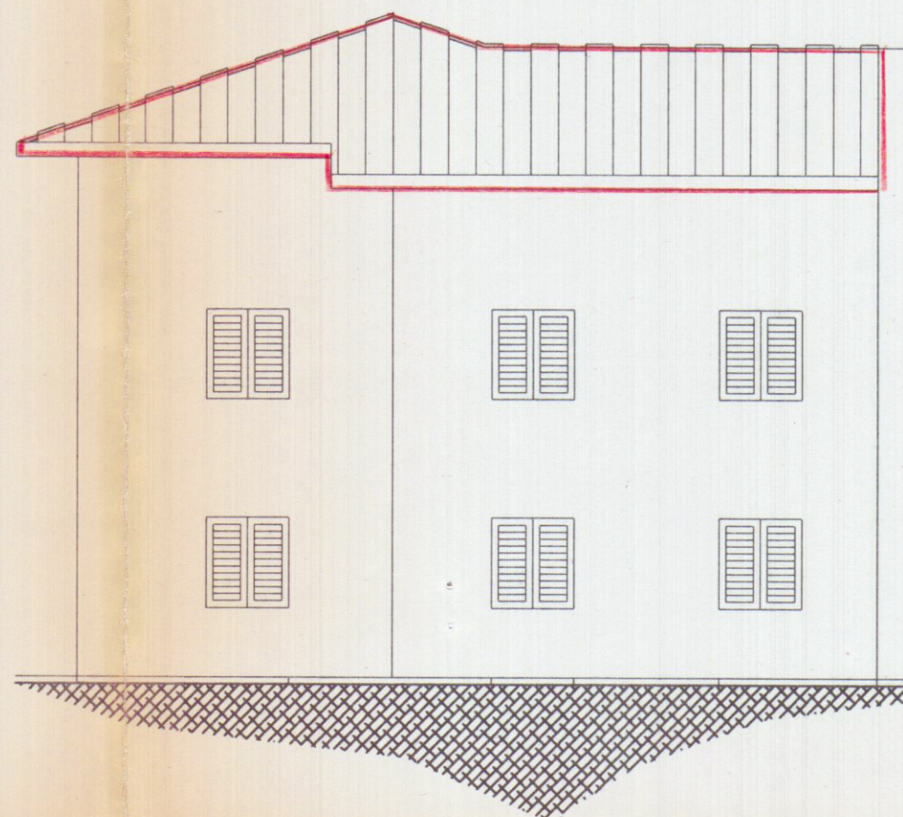
PROSPETTO NORD
