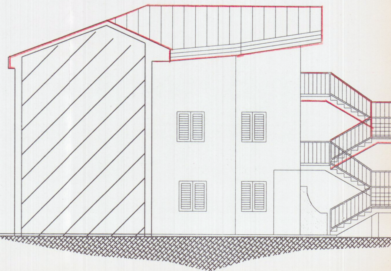
PROSPETTO OVEST
