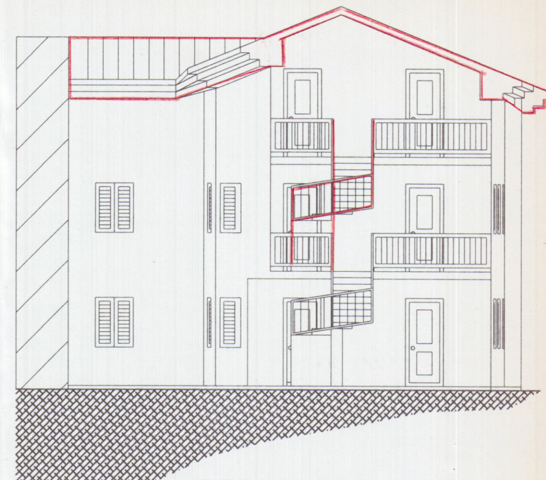
PROSPETTO SUD
