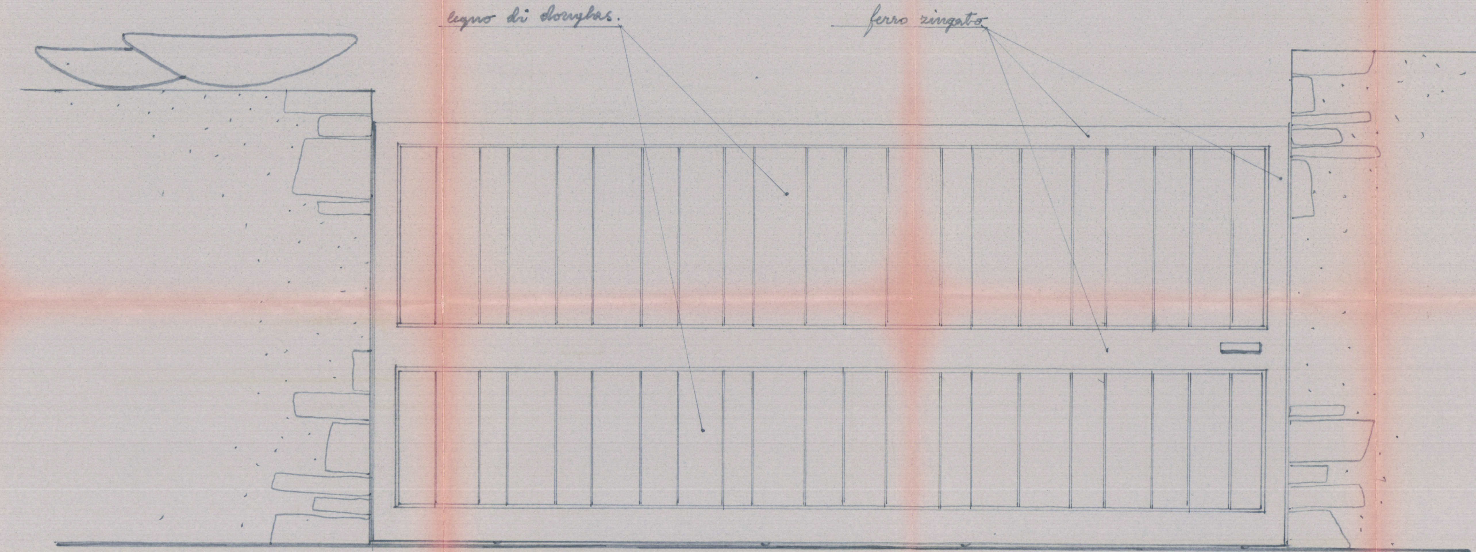
PARTICOLARE 1:10. CANCELLO SCORREVOLE
