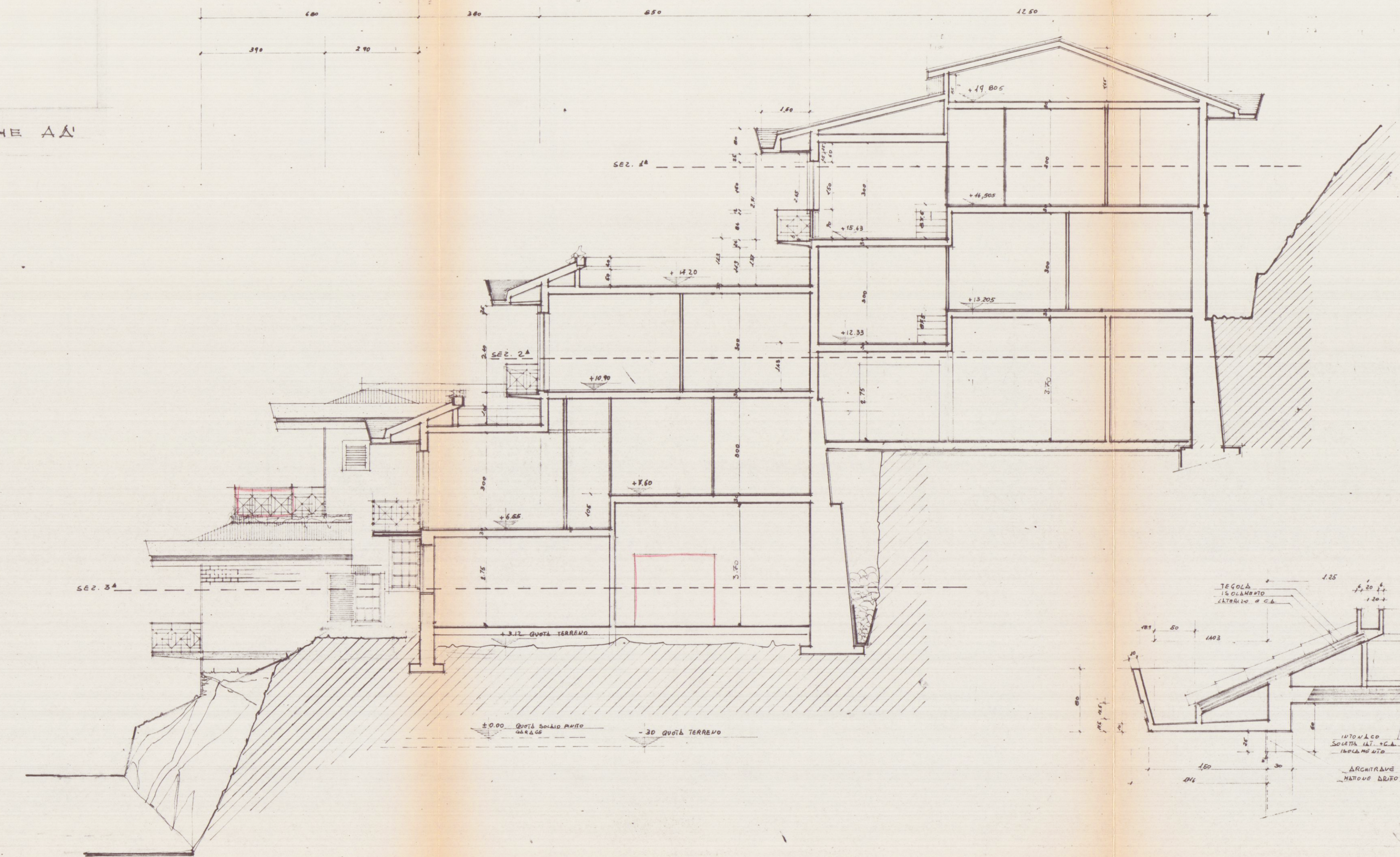
PROSPETTO SUB-EST TAV. 8
